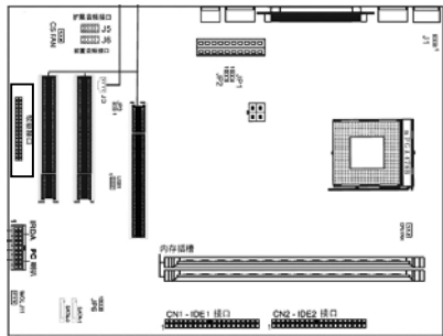
图 25 FDD 软驱接口
