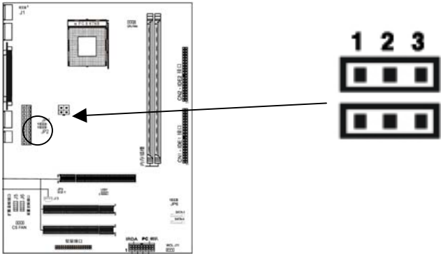
JP1 和 JP2:CPU 频率跳线设置
