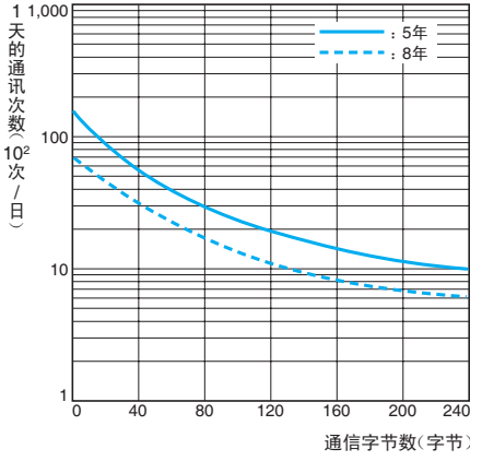
V600-D8KR13电池寿命特性
