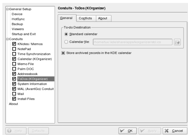
圖形 6.3 顯示 KOrganizer 行事曆檔案路徑的對話方塊
