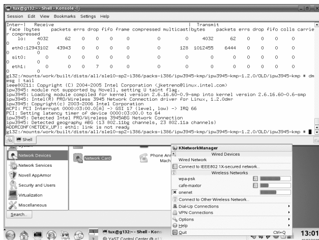
圖形 13.1 KNetworkManager Applet 中可用的網路
