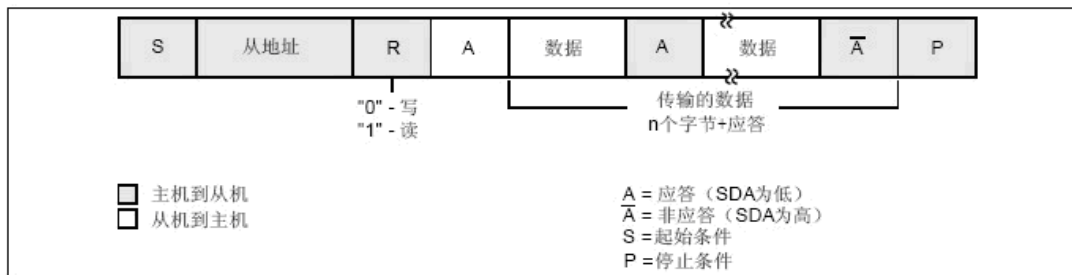
主接收器模式的格式
