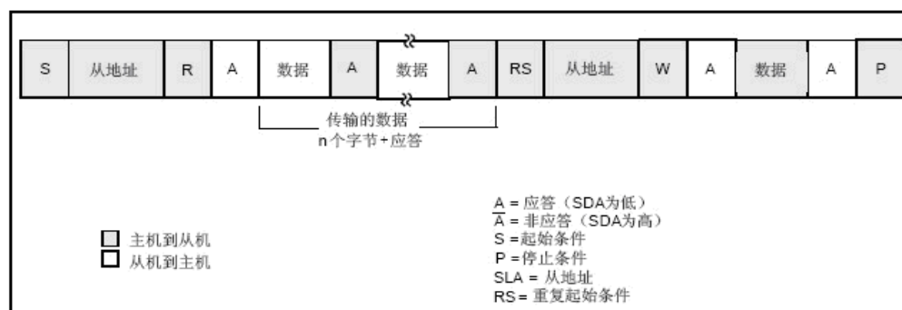
在发送重复起始条件后，主接收器切换到主发送器
