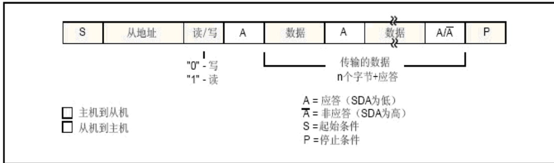
主发送器模式中的格式
