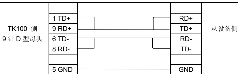
MD2-MODBUS-RS422 连线图
