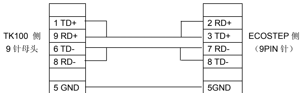
MD-ECOSTEP-CAB422 连线图
