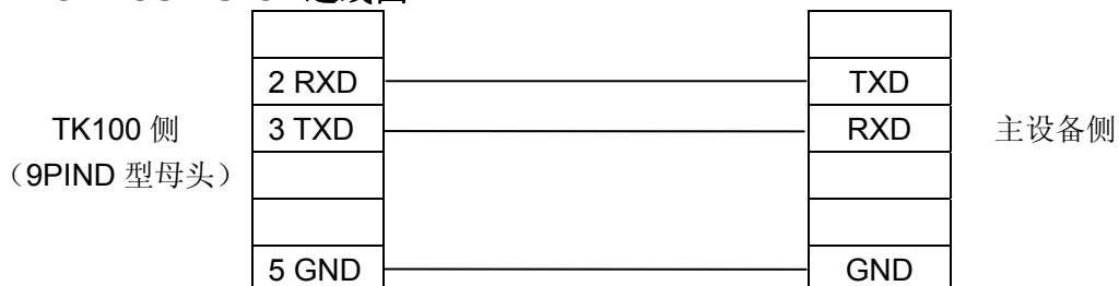
MD2-MODBUS-RS485 连线图
