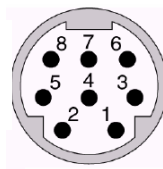
8 针圆形母座管脚图 (注意公头管脚左右顺序相反)
