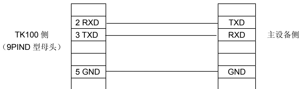
MD2-FREEPTC-RS232 连线图
