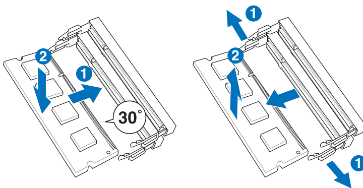
安装内存模块
