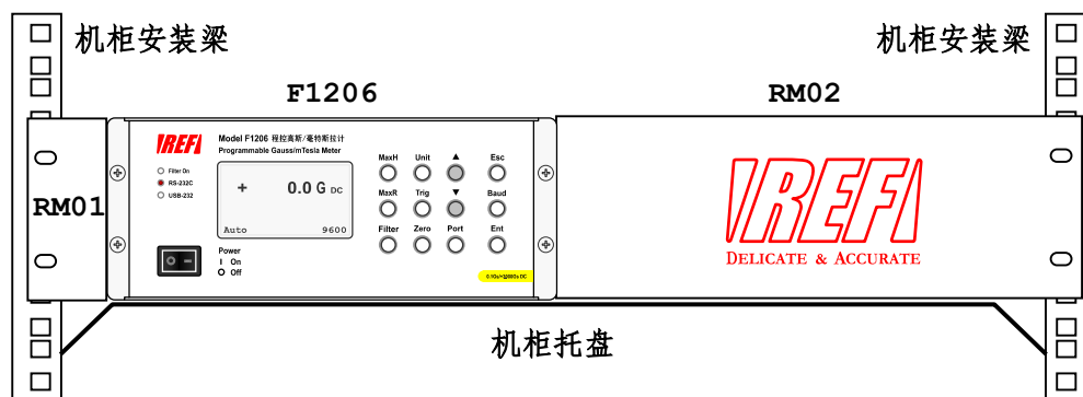
图 2-5 F1206 与机柜的连接安装方法
