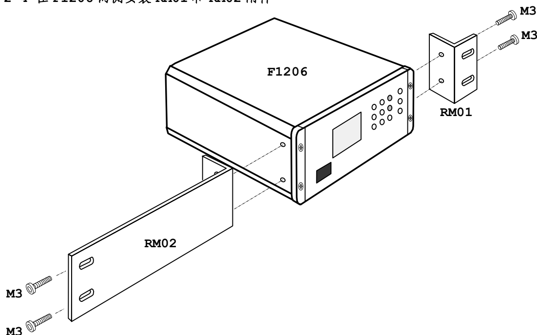
图 2-4 在 F1206 两侧安装 RM01 和 RM02 附件
