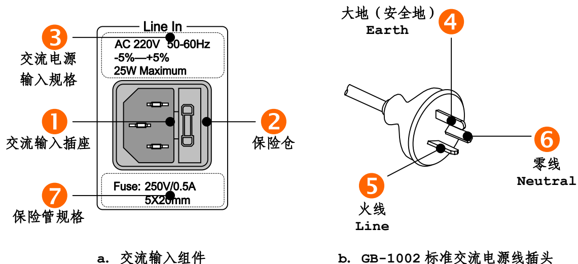
图 2-7 电源输入组件和交流电源线插头
