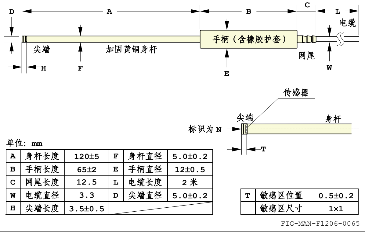
图 5-2 F12004 通用数字化轴向霍尔探头二视图
