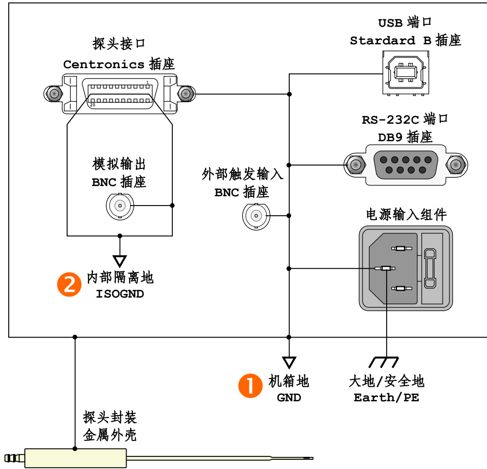
图 3-41 F1206 的接地关系
