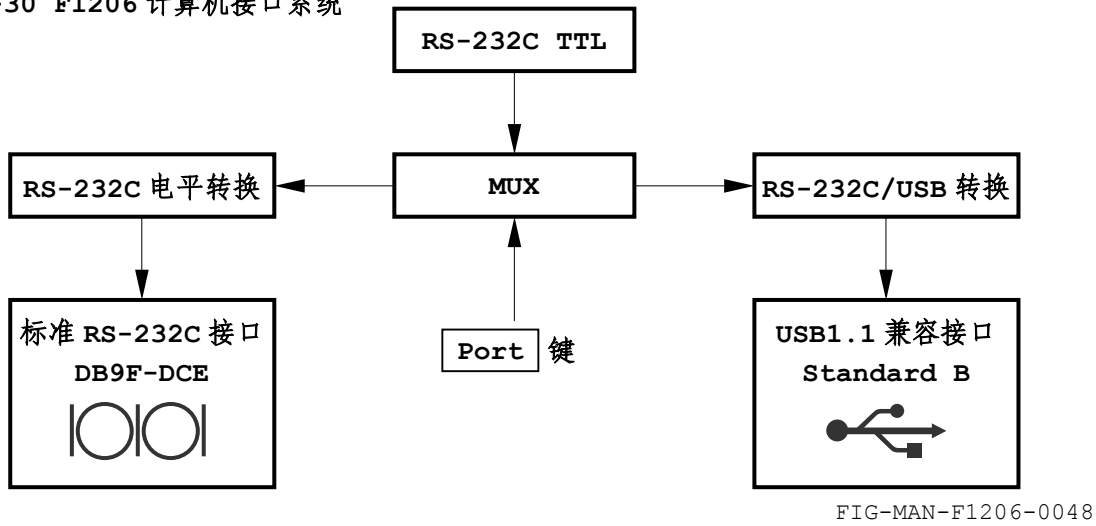
图 3-30 F1206 计算机接口系统
