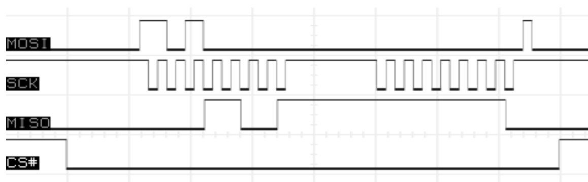
图7. 工作在(1,1)模式下的SPI接口
