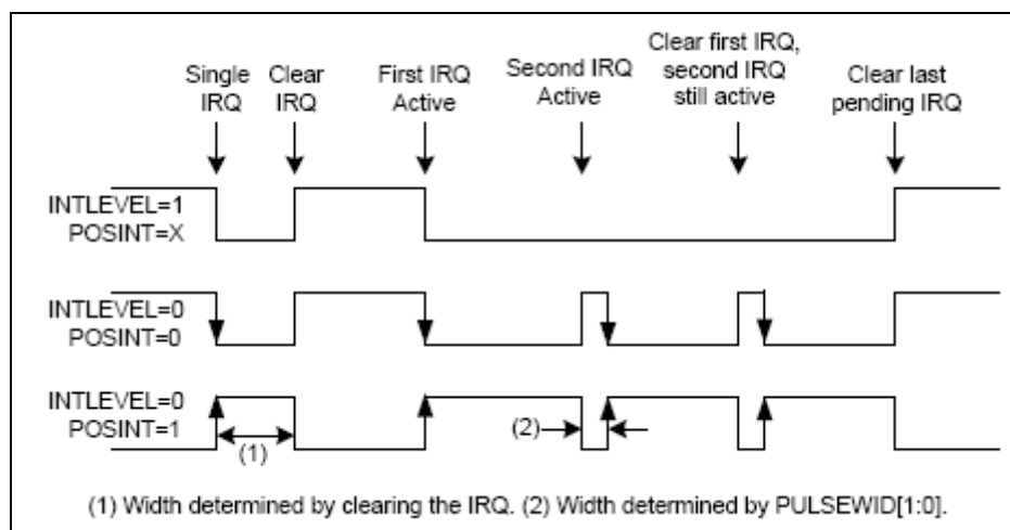
图8. INT 引脚的动作取决于INTLEVEL 位和POSINT 位
