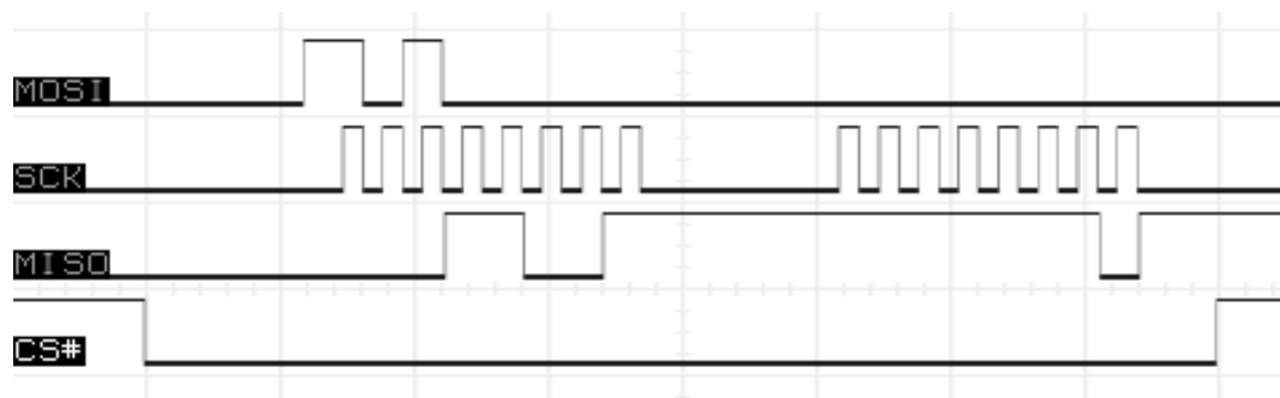
图6. 工作在(0,0)模式下的SPI接口
