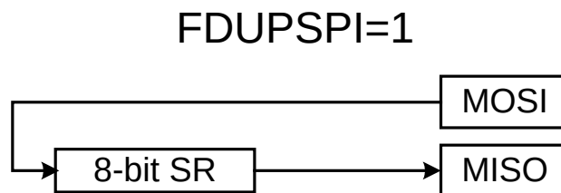
图4. 全双工SPI接口
