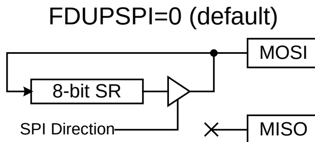
图3. 半双工SPI接口
