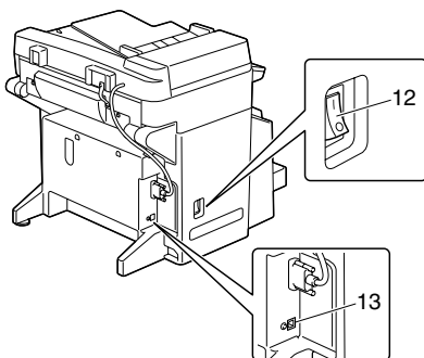
(后视图)
