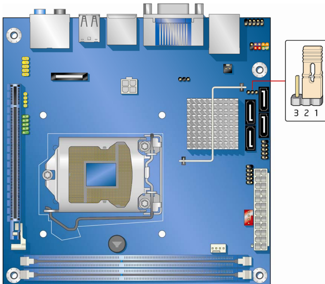
图 24. BIOS 配置跳线块位置
