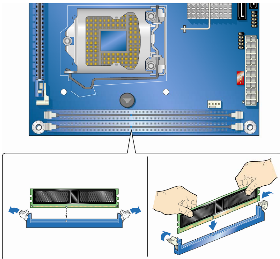
图 16. 安装 DIMM
