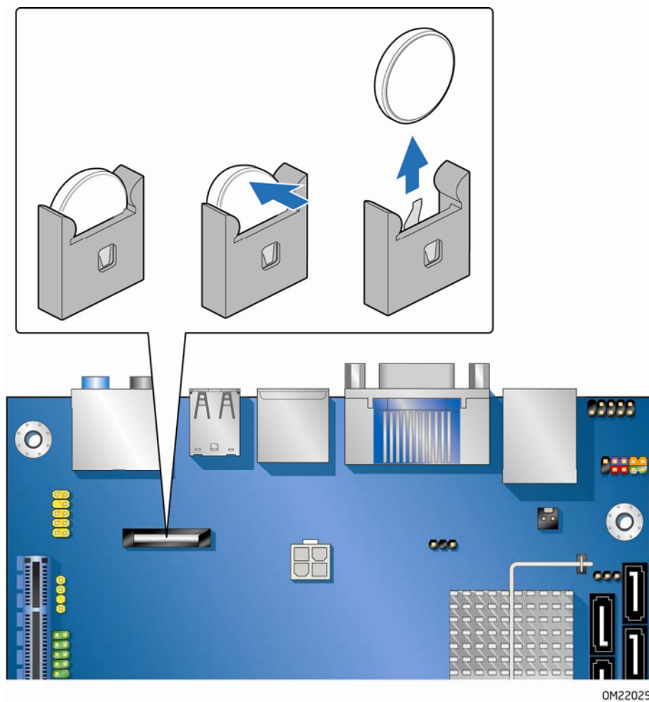
图 25. 拆卸电池
