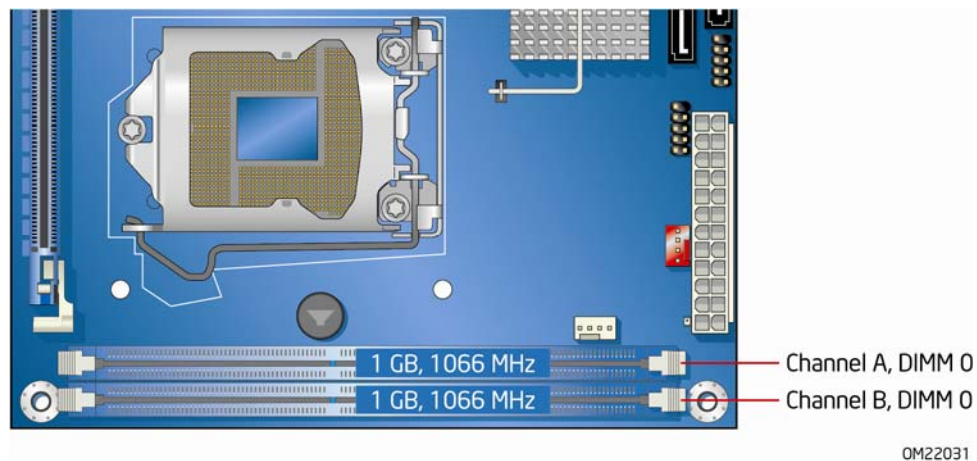
图 14. 双通道内存配置示例
