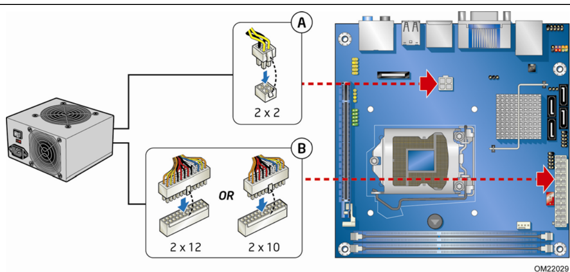
图 23. 连接电源系统电缆
