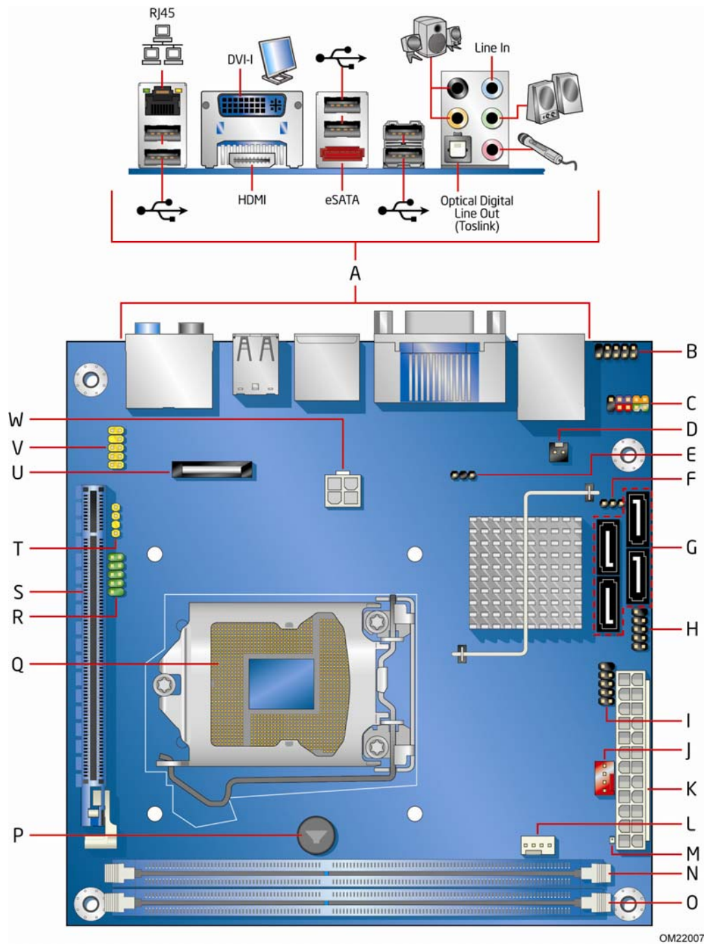
图 1. 英特尔台式机主板 DH57JG 组件
