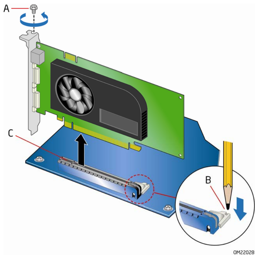
图 18. 拆卸 PCI Express x16 图形卡
