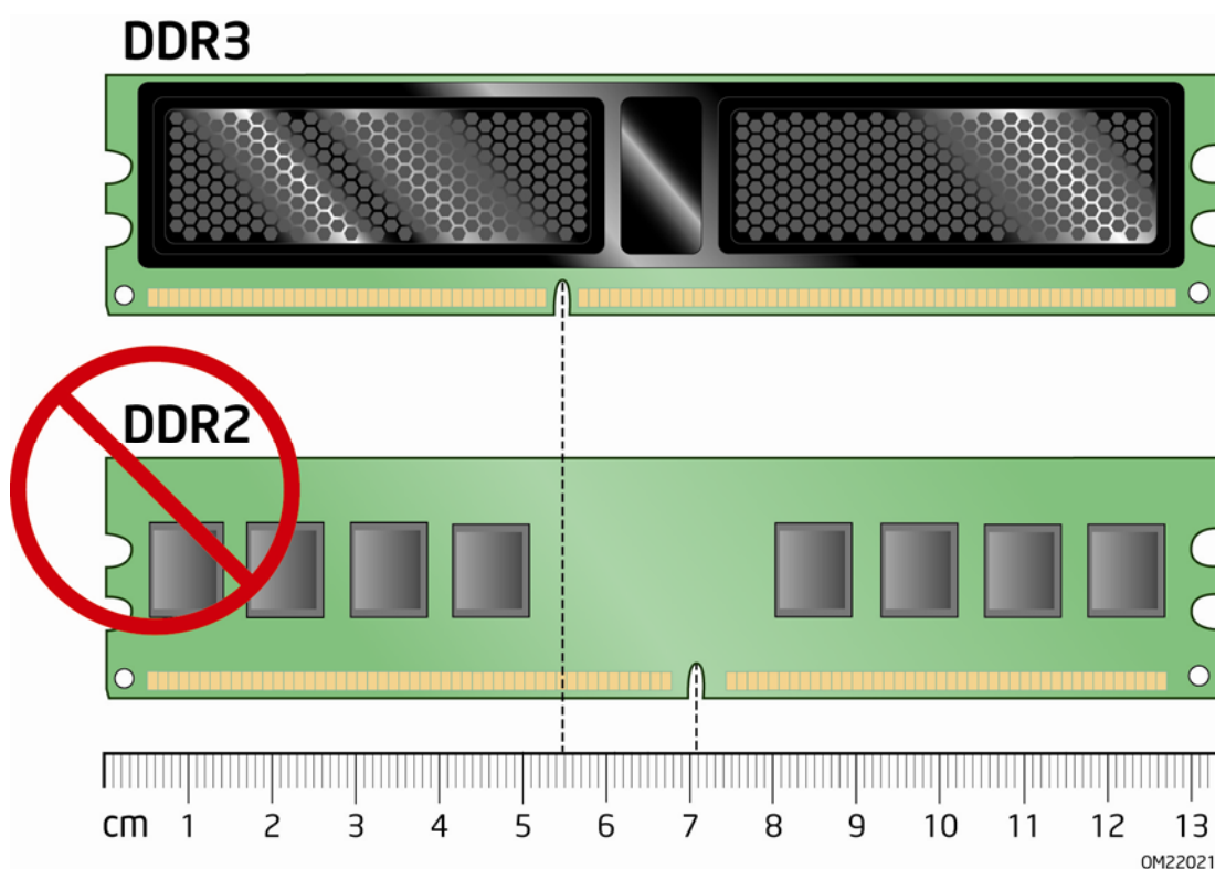
图 15. 使用 DDR3 DIMM
