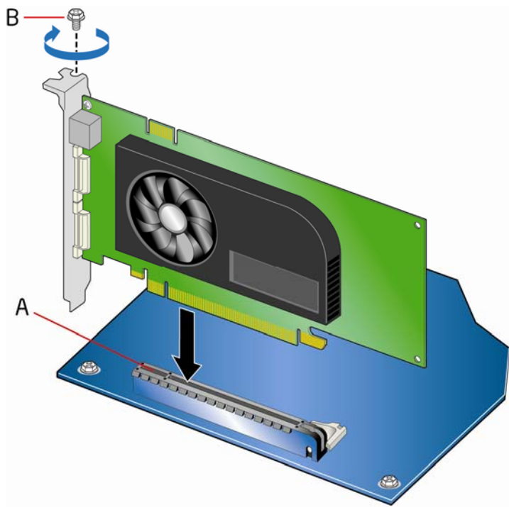
图 17. 安装 PCI Express x16 图形卡
