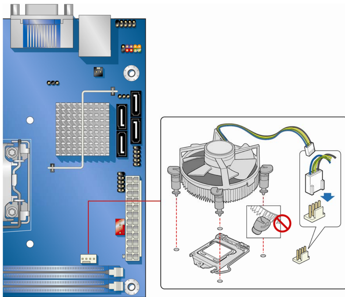
图 13. 将处理器风扇散热器电源电缆连接到处理器风扇接头连接器上
