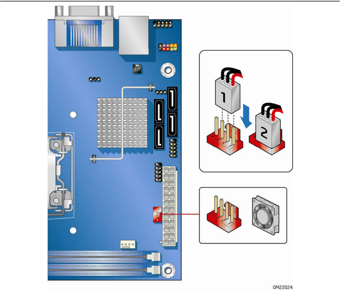
图 22. 机箱风扇接头连接器位置
