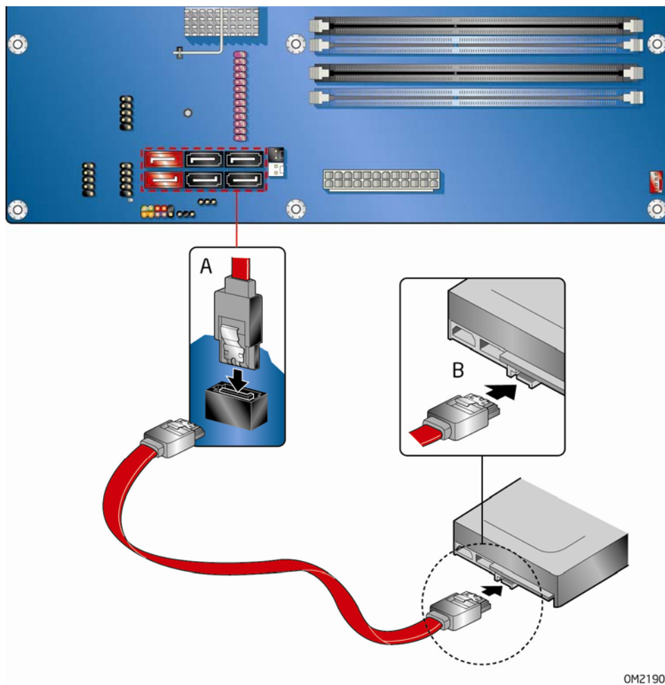
图 19. 连接串行 ATA 电缆
