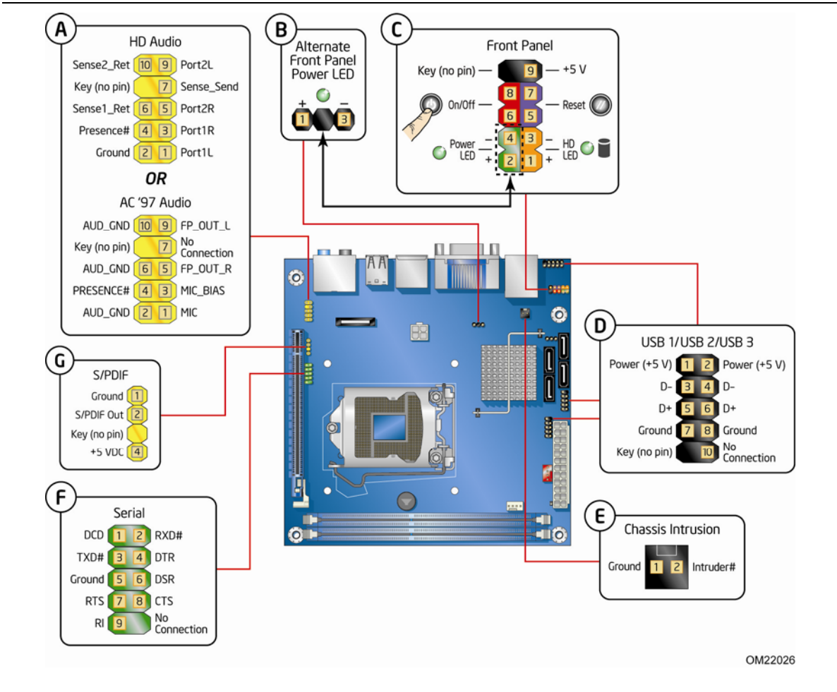
图 20. 内置接头连接器
