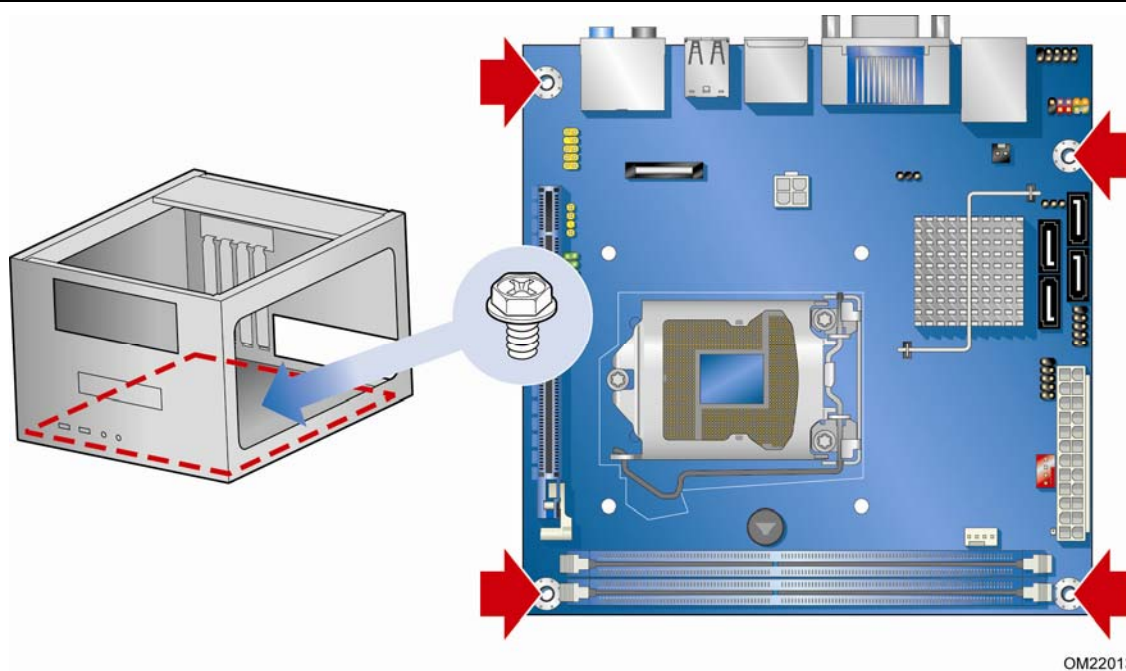
图 5. 英特尔台式机主板 DH57JG 安装螺丝孔位置
