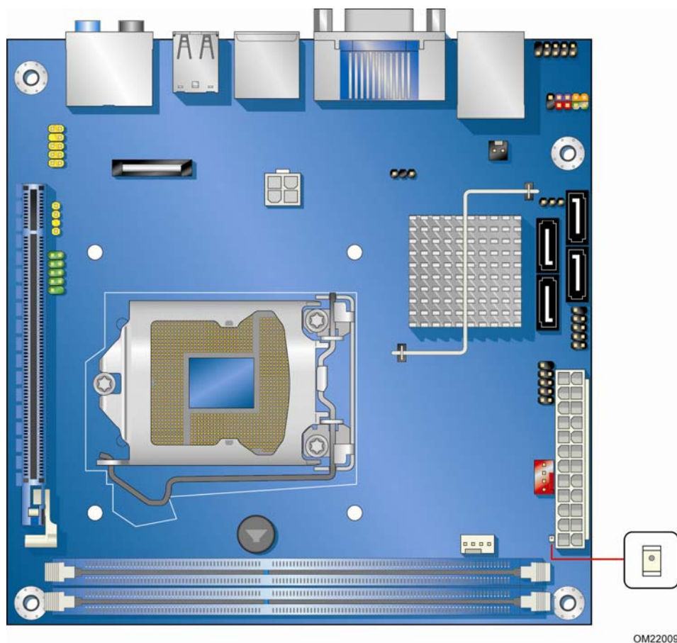
图 3. 备用电源指示灯位置
