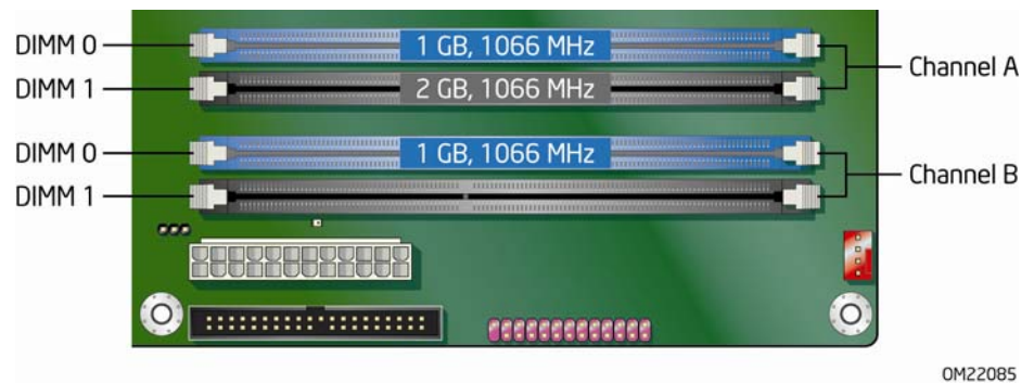
图 15. 三条 DIMM 下双通道内存配置
