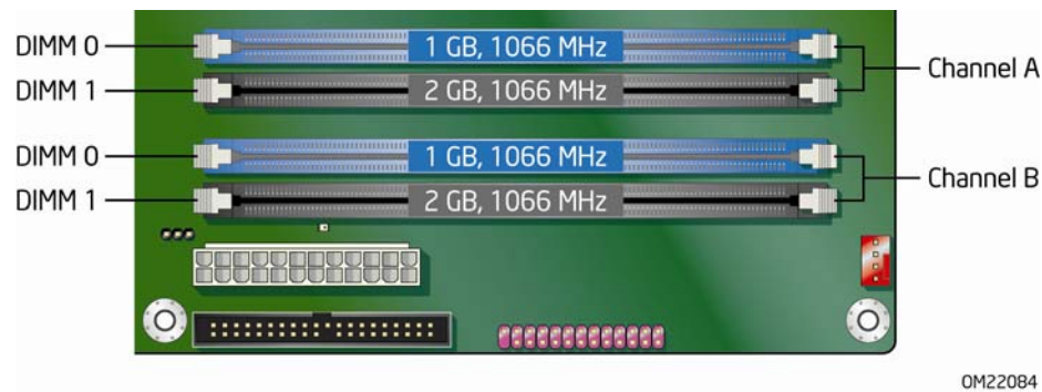
图 14. 四条 DIMM 下双通道内存配置
