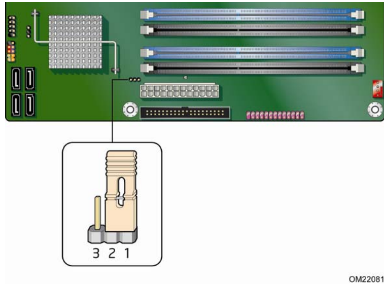
图 26. BIOS 配置跳线块位置
