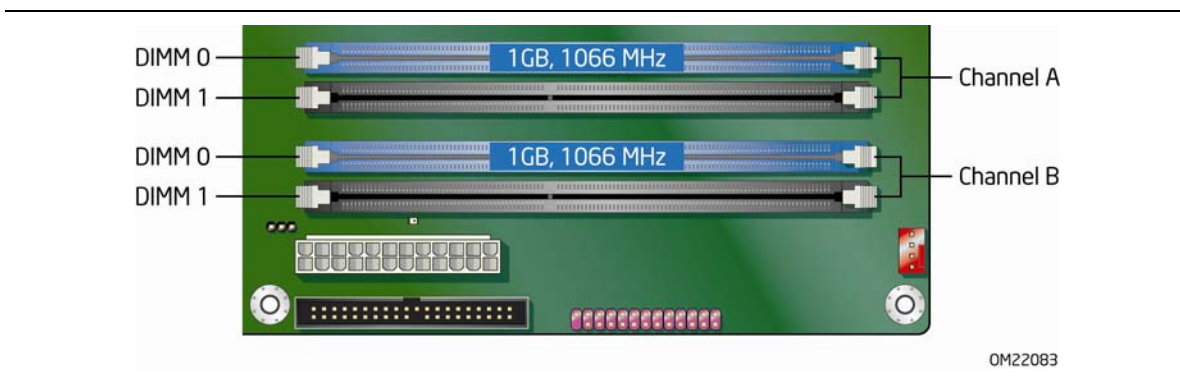
图 13. 两条 DIMM 下双通道内存配置
