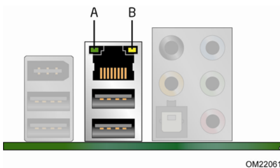
图 2. LAN 状态 LED 指示灯
