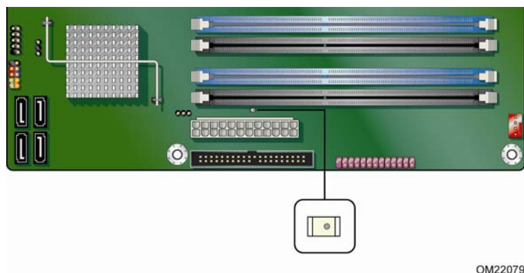
图 3. +5 V 备用电源指示灯位置
