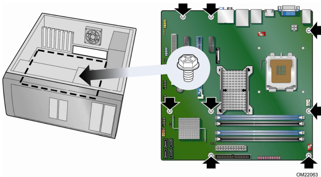
图 5. 英特尔台式机主板 DG43RK 安装螺丝孔位置
