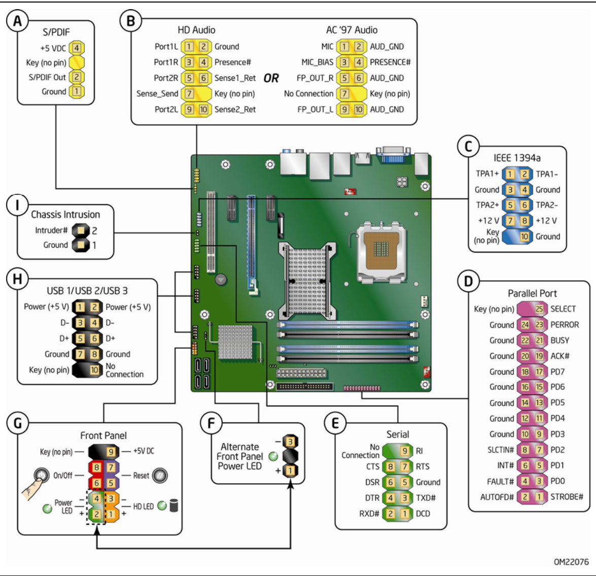
图 22. 内置接头连接器
