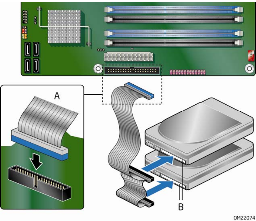
图 20. 连接 IDE 电缆
