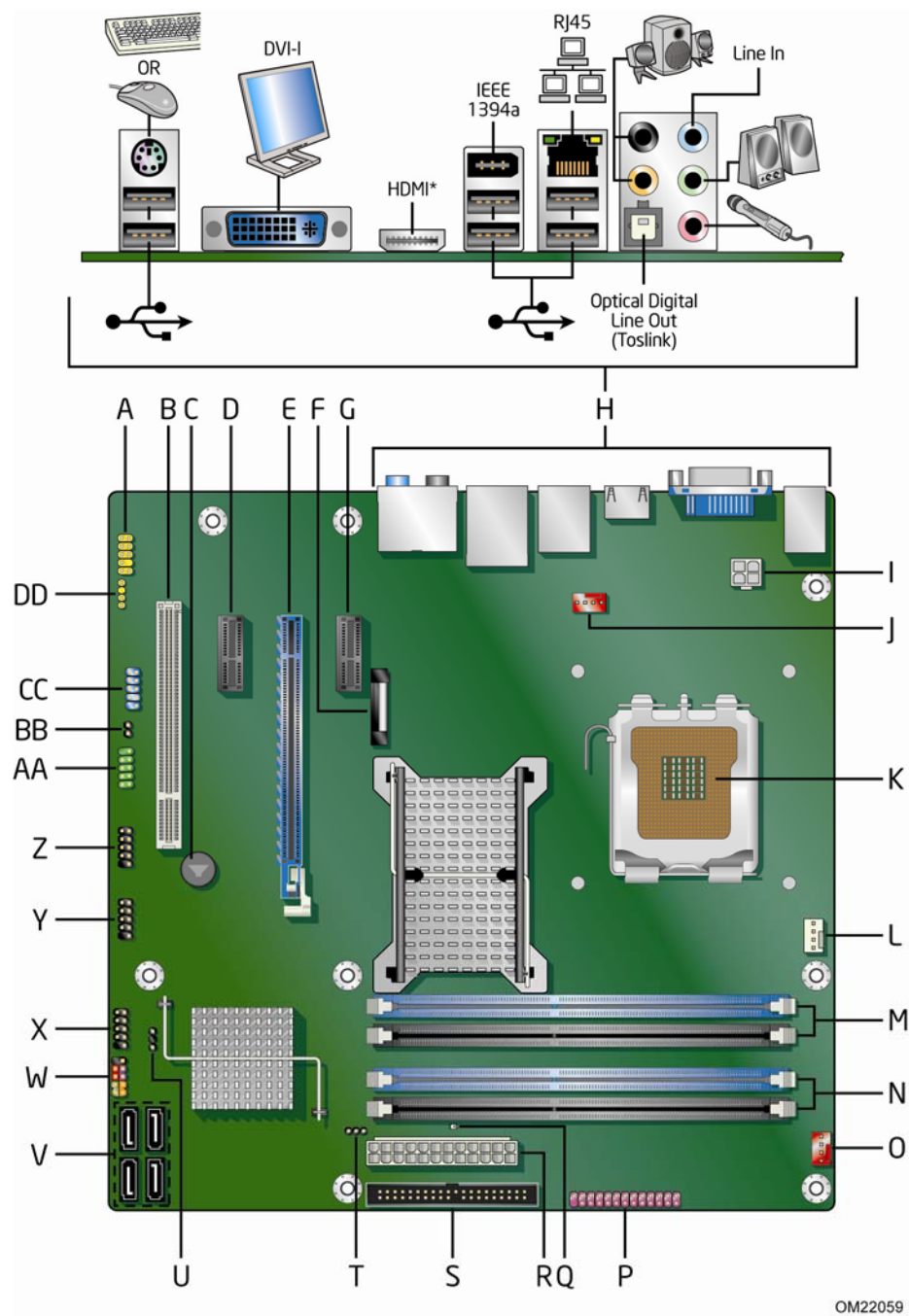
图 1. 英特尔台式机主板 DG43RK 组件
