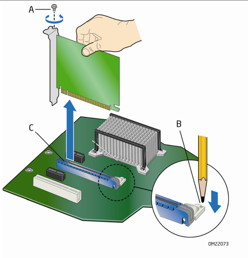
图 19. 拆卸 PCI Express x16 卡
