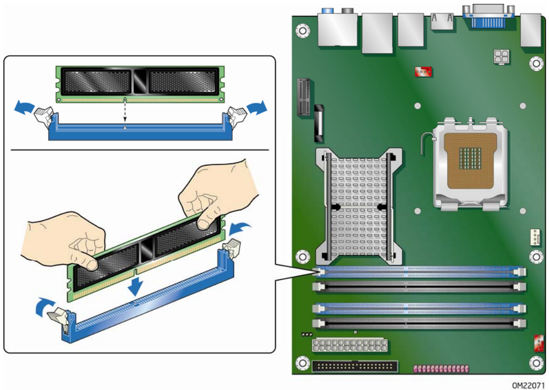
图 17. 安装 DIMM
