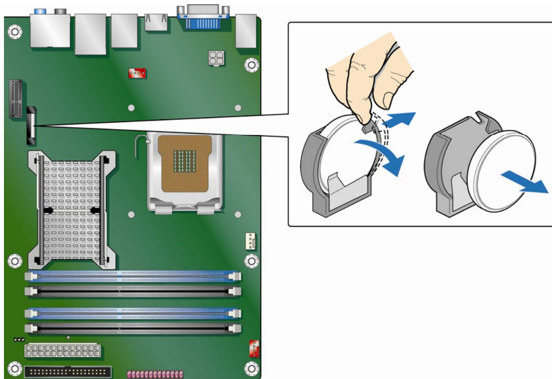
图 27. 拆卸电池
