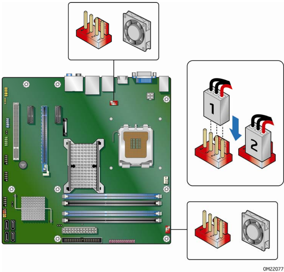
图 24. 机箱风扇接头连接器位置
