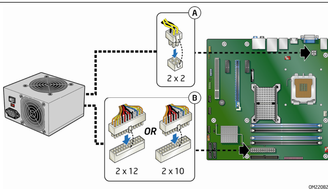
图 25. 连接电源系统电缆
