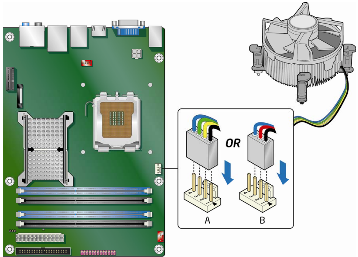
图 12. 连接处理器风扇散热器电缆
