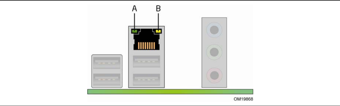
图 2. LAN 连接器 LED 指示灯
