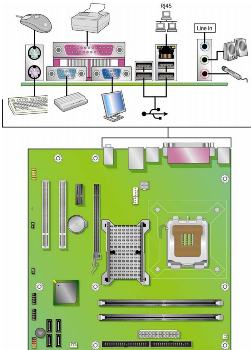
图 26. 背面板连接器
