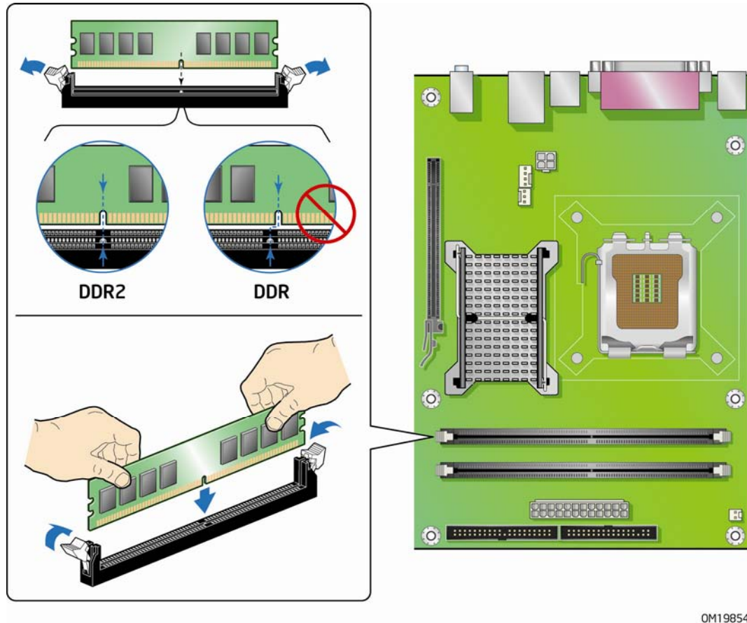
图 15. 安装 DIMM
