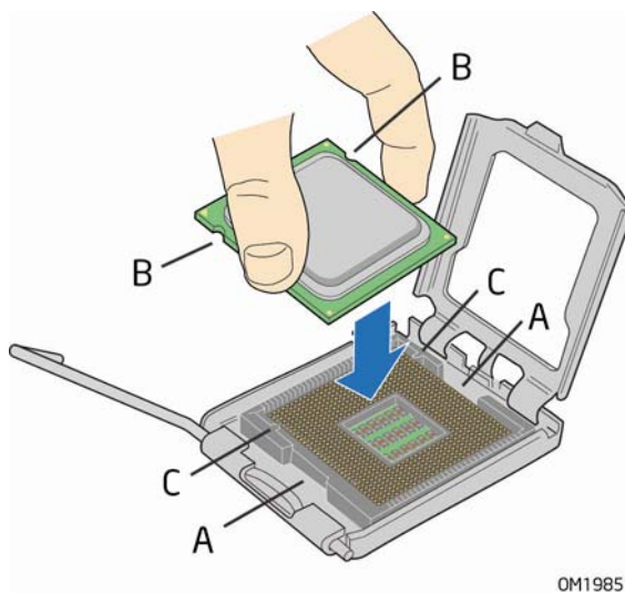
图 10. 安装处理器
