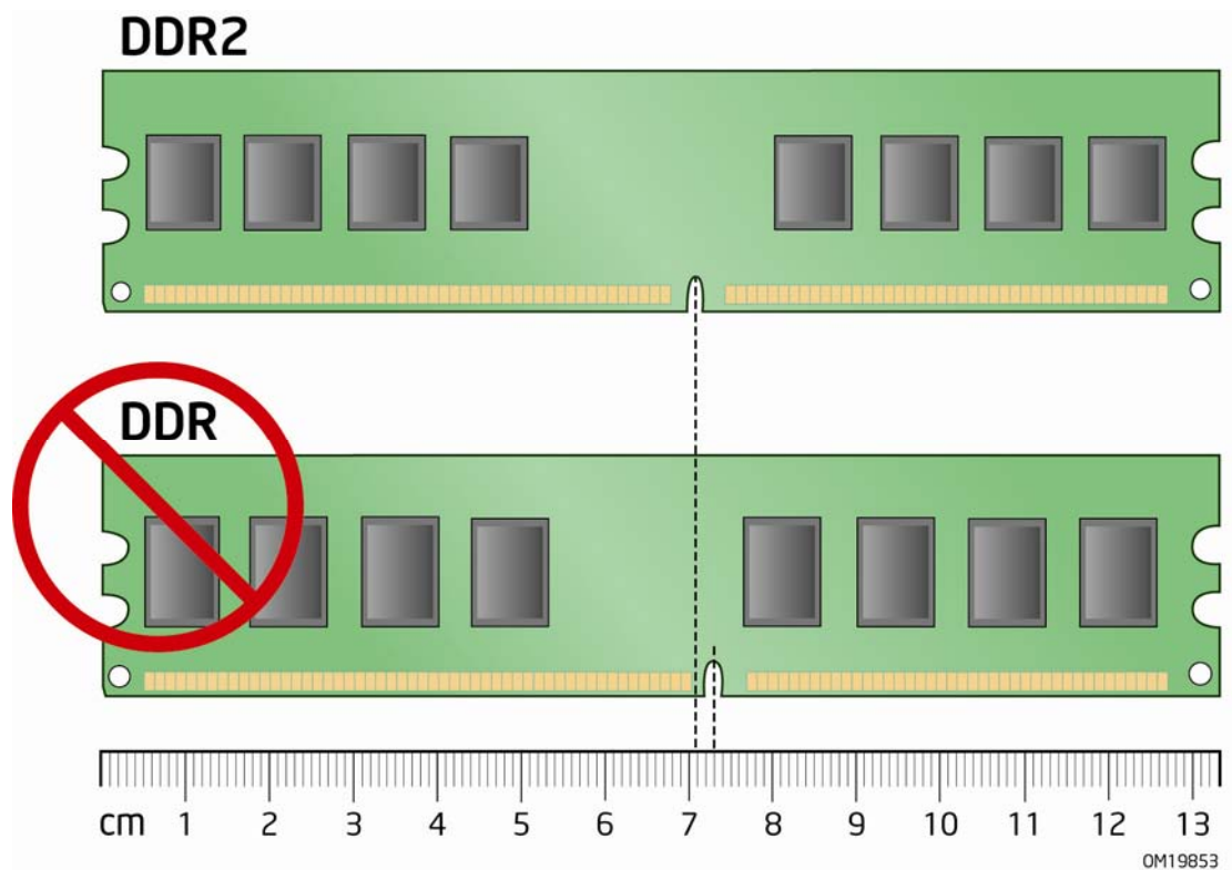
图 14. 使用 DDR2 DIMM
