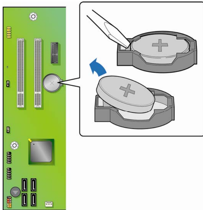
图 27. 拆卸电池
