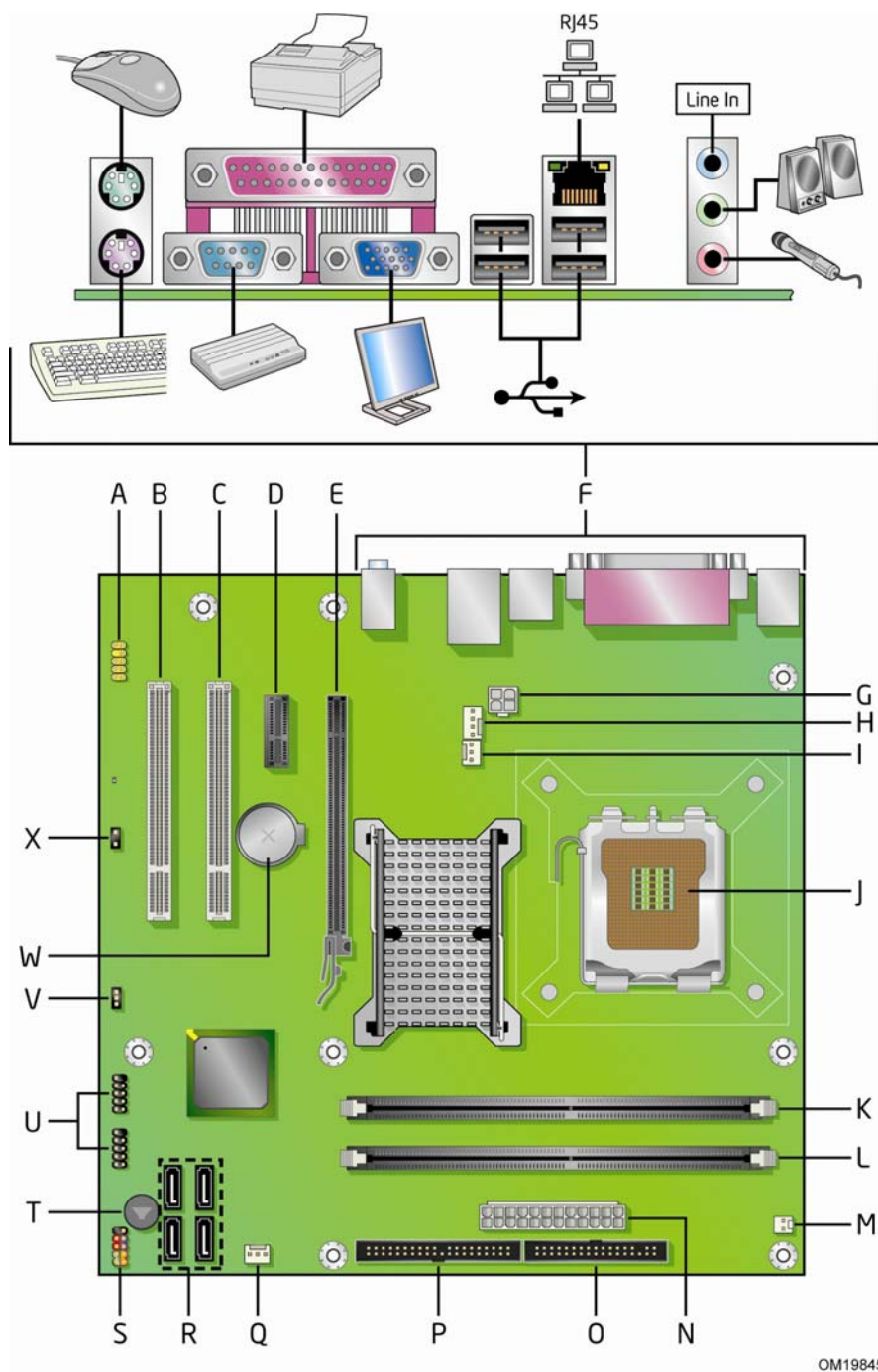
图 1. 台式机主板 D945GCCR 组件
