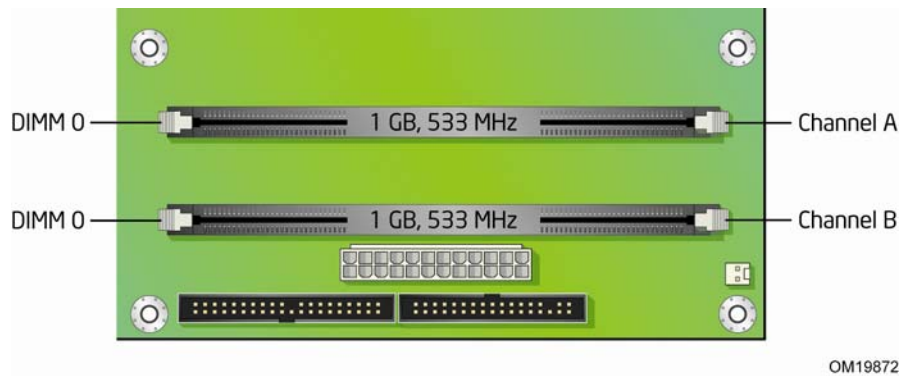
图 13. 双通道内存配置示例
