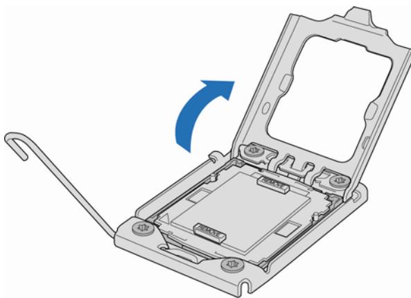
图 10. 抬起压板
