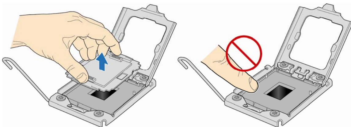
图 11. 拆卸插槽保护罩
