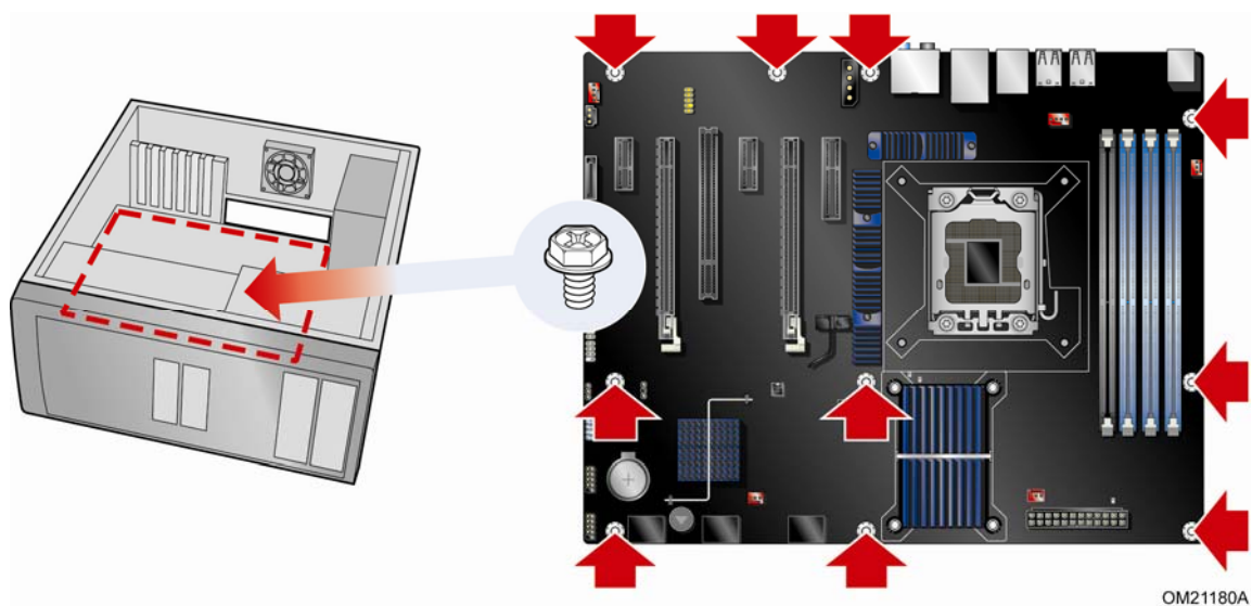
图 8. 英特尔台式机主板 DX58SO 安装螺丝孔位置
