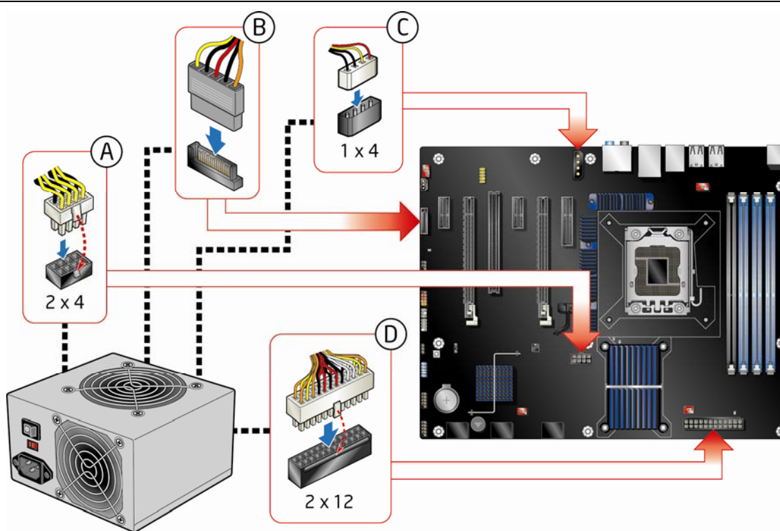
图 30. 连接电源系统电缆
