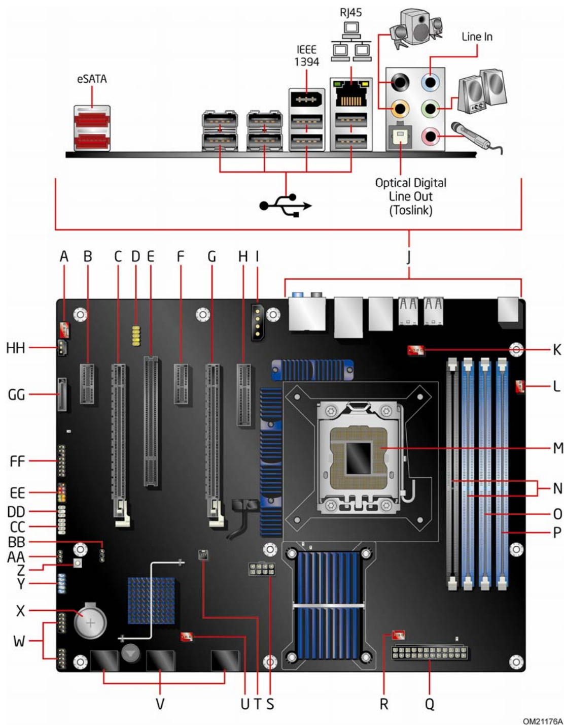
图 1. 英特尔台式机主板 DX58SO 组件
