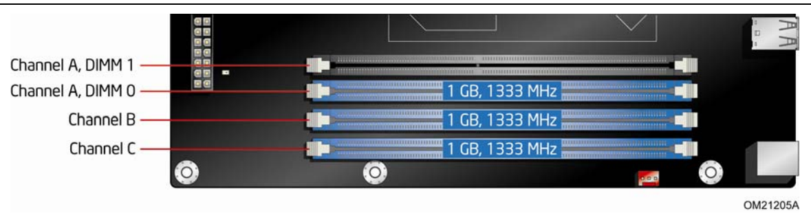
图 18. 三通道内存配置
