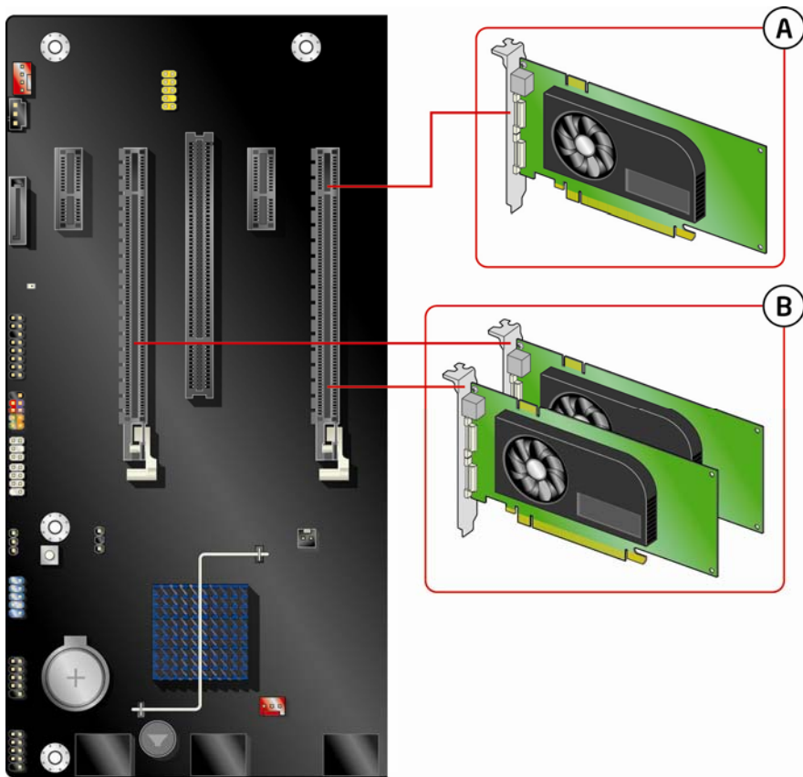
图 23. 安装 PCI Express x16 图形卡
