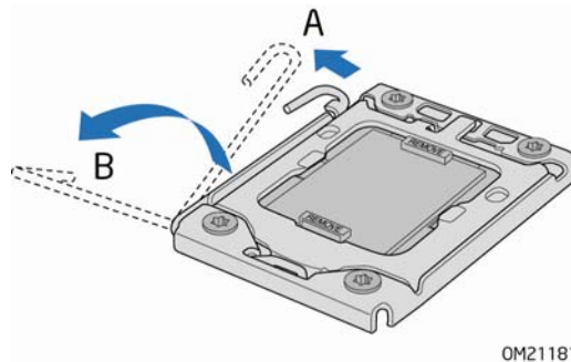
图 9. 抬起插槽拉杆
