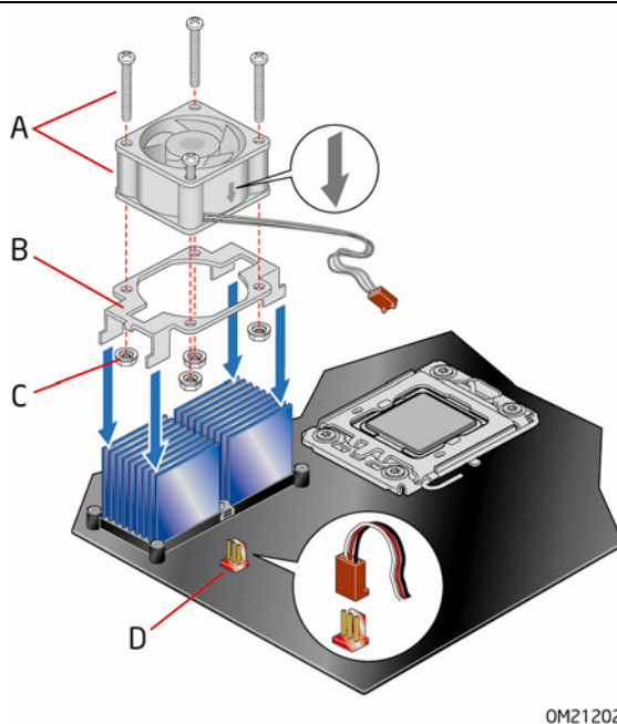
图 17. 安装 IOH 风扇
