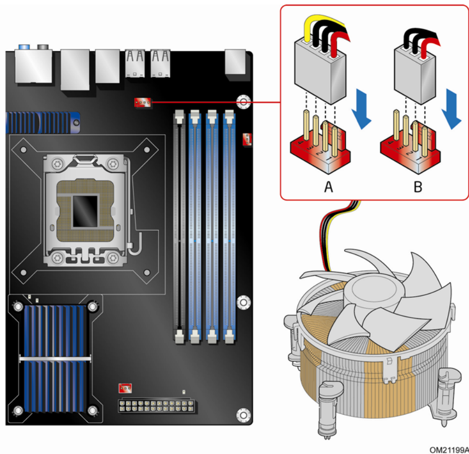
图 15. 将处理器风扇散热器电缆连接到处理器风扇接头连接器上
