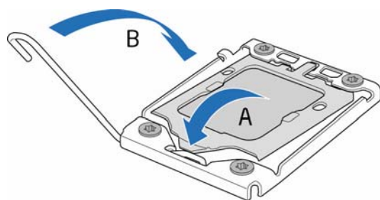
图 14. 闭合压板
