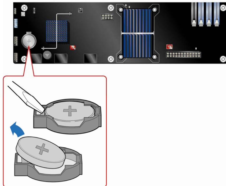
图 32. 拆卸电池
