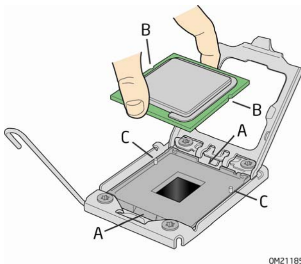
图 13. 安装处理器
