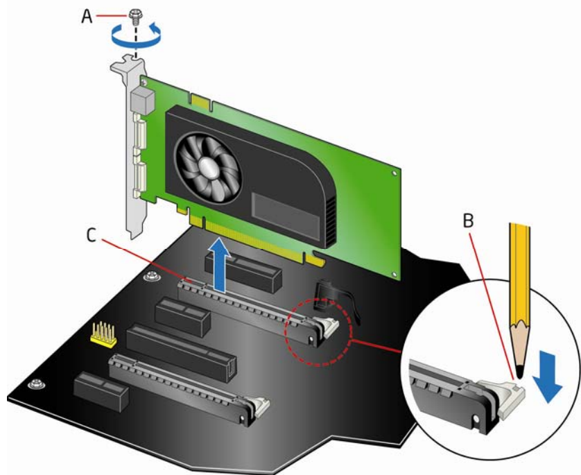
图 25. 拆卸 PCI Express x16 卡
