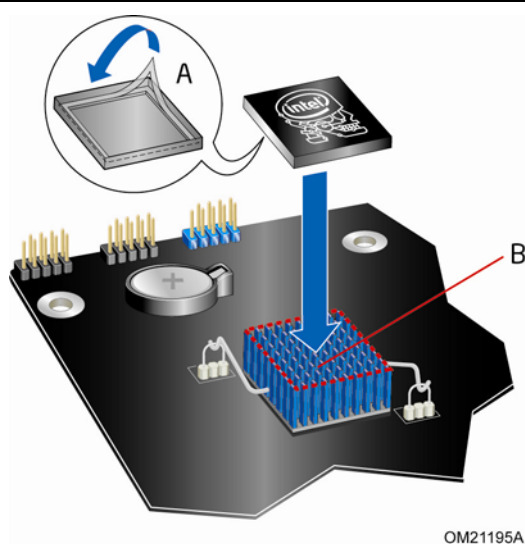
图 16. 安装 ICH 散热器装饰罩
