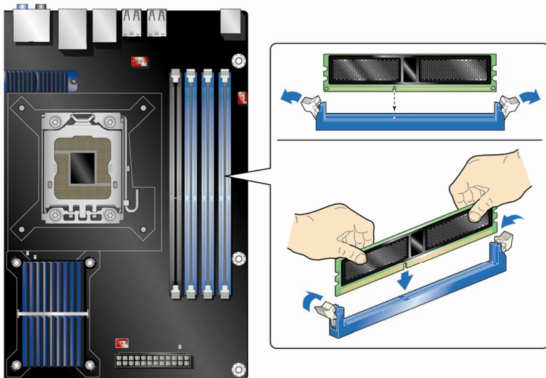
图 22. 安装 DIMM
