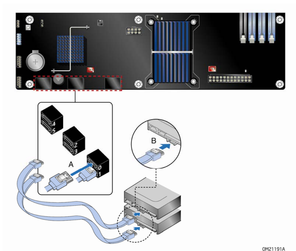
图 26. 连接串行 ATA 电缆
