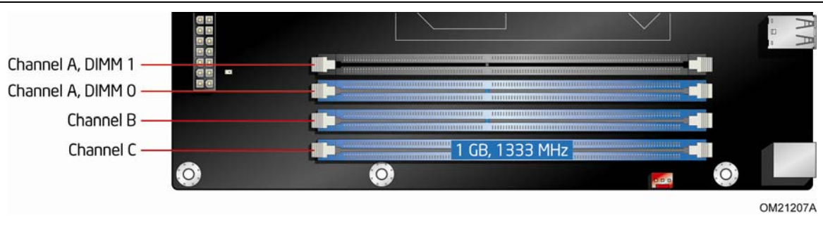
图 20. 单通道内存配置
