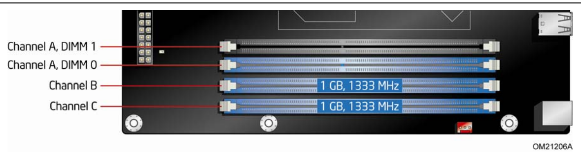
图 19. 双通道内存配置
