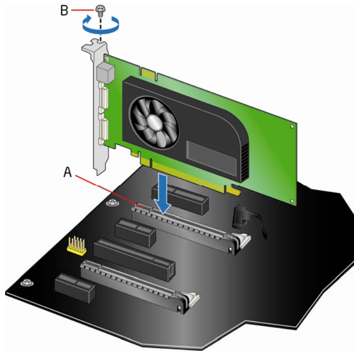
图 24. 安装 PCI Express x16 卡
