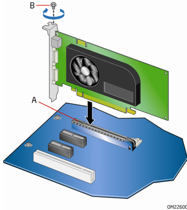
图 17. 安装 PCI Express x16 图形卡
