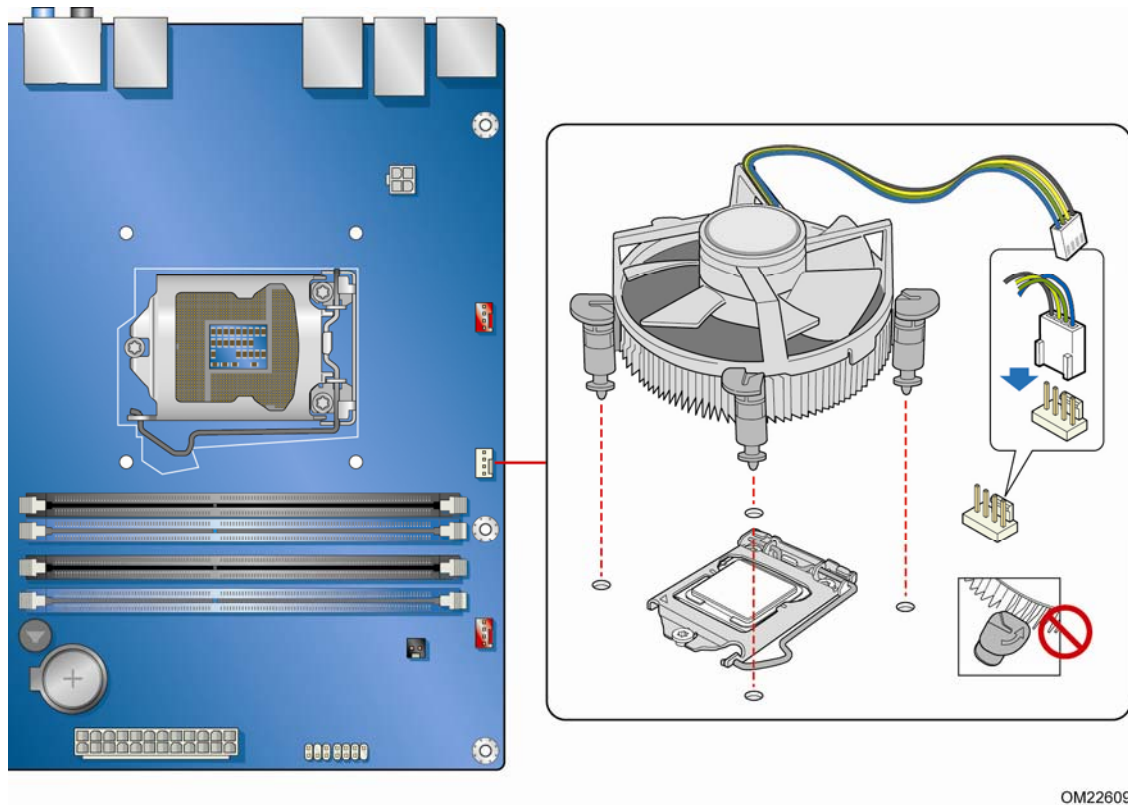
图 11. 将处理器风扇散热器电源电缆连接到处理器风扇接头连接器上
