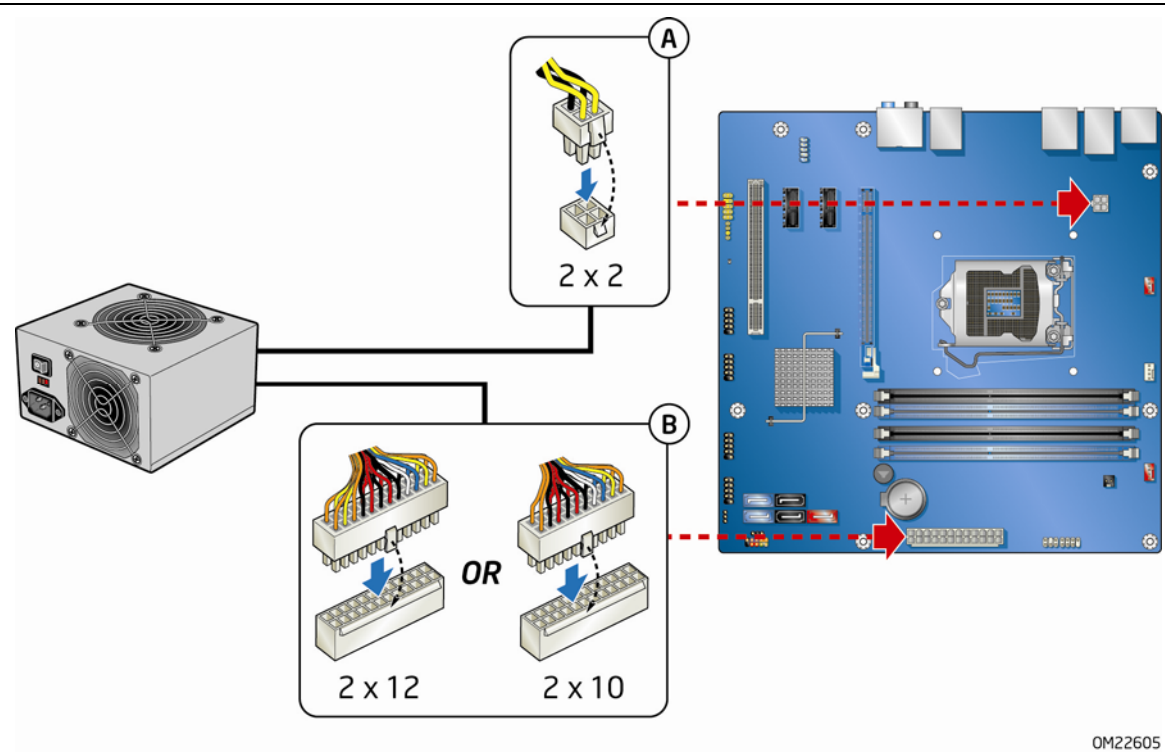
图 23. 连接电源系统电缆
