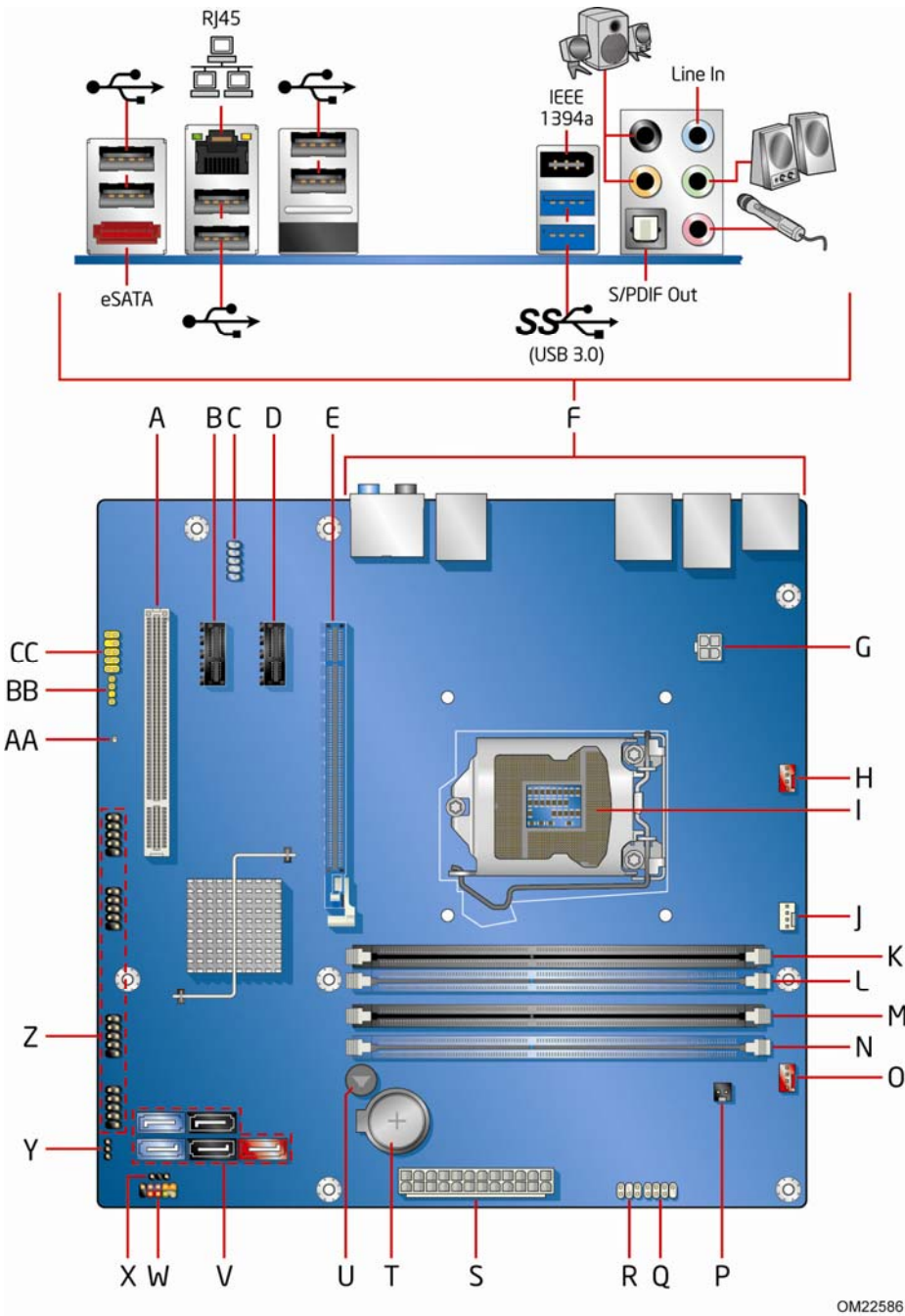
图 1. 英特尔台式机主板 DP67DE 组件
