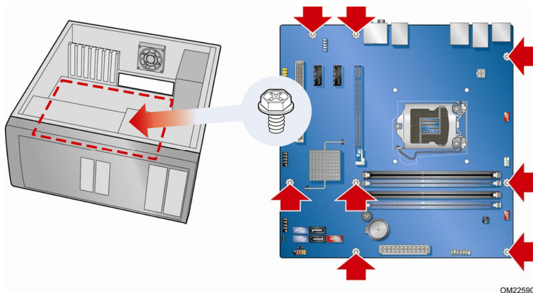
图 5. 英特尔台式机主板 DP67DE 安装螺丝孔位置
