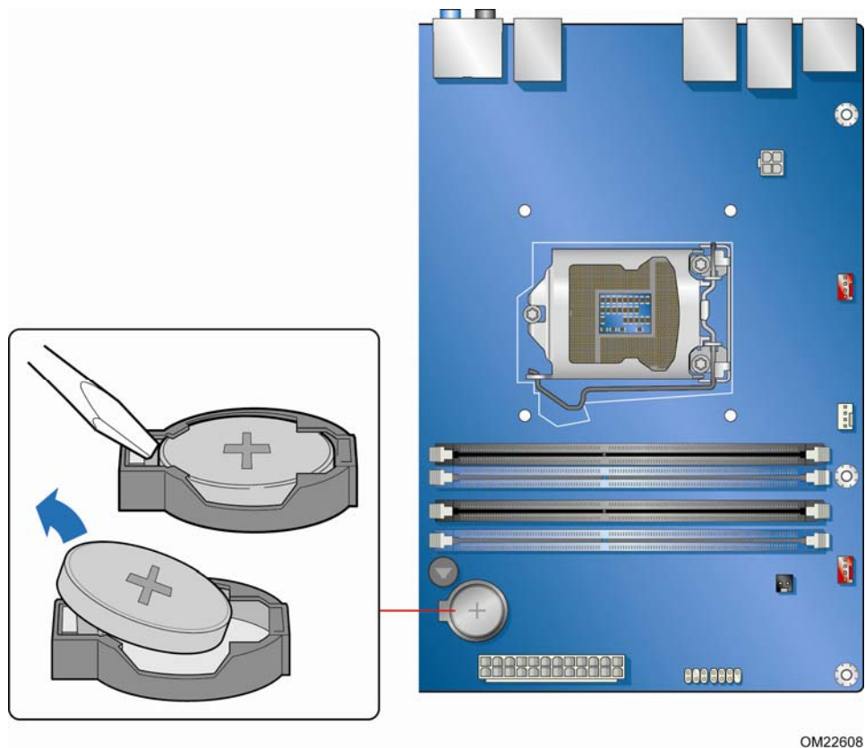
图 25. 拆卸电池
