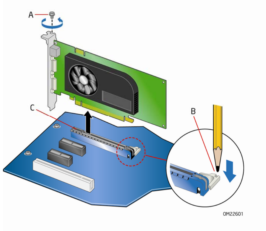
图 18. 拆卸 PCI Express x16 图形卡
