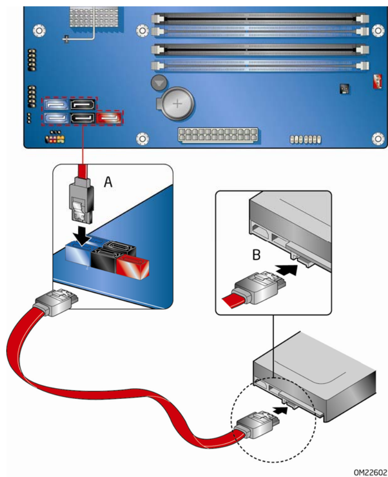
图 19. 连接 SATA 驱动器
