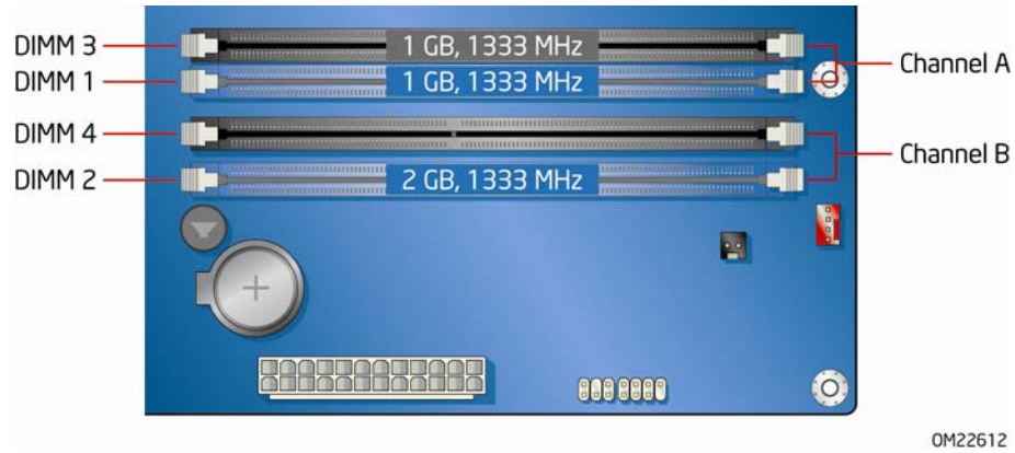
图 14. 三条 DIMM 下双通道内存配置示例
