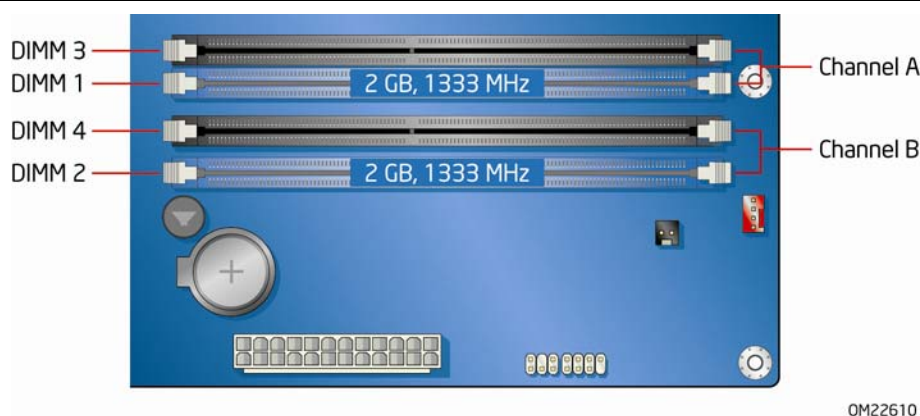
图 12. 两条 DIMM 下双通道内存配置示例
