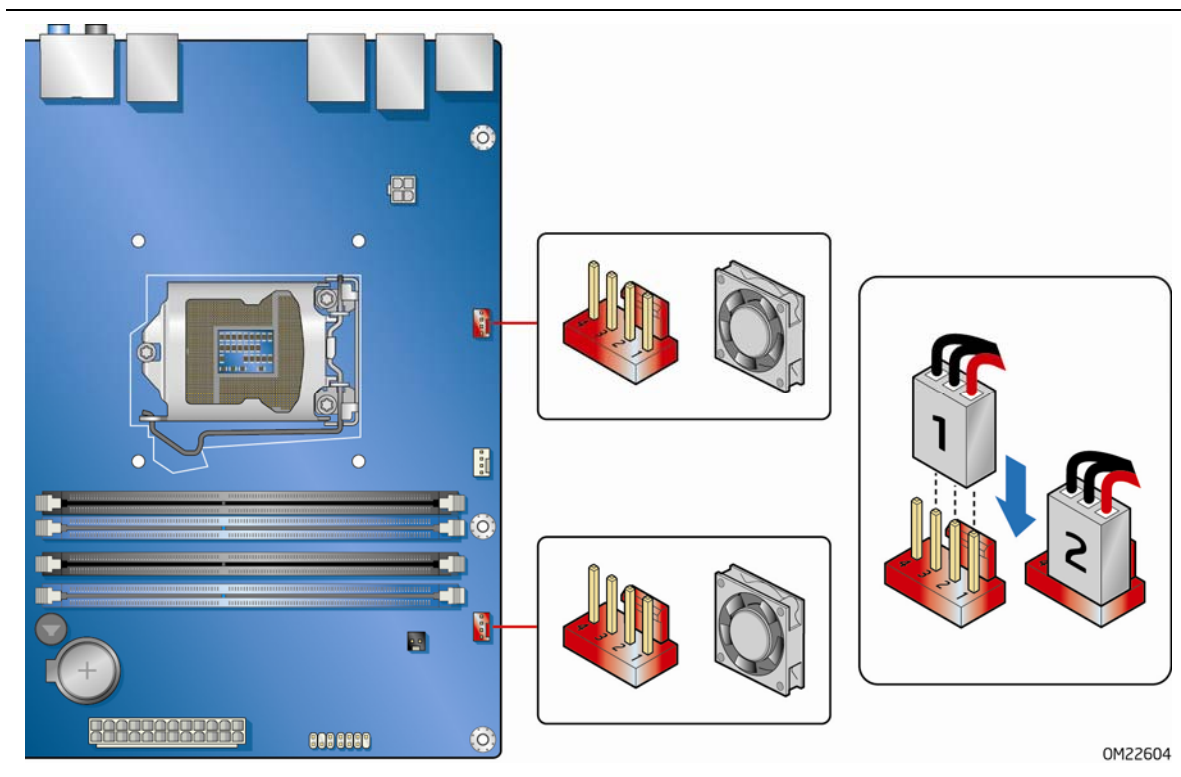
图 22. 机箱风扇接头连接器位置
