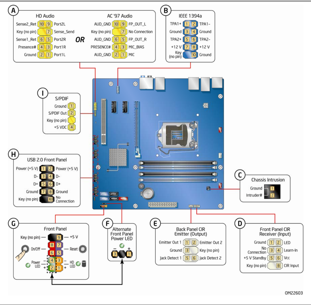
图 20. 内置接头连接器
