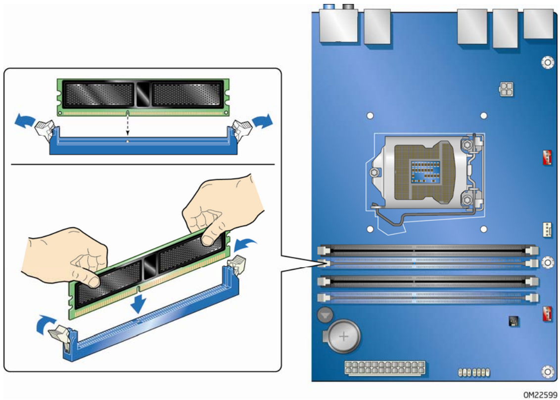
图 16. 安装 DIMM
