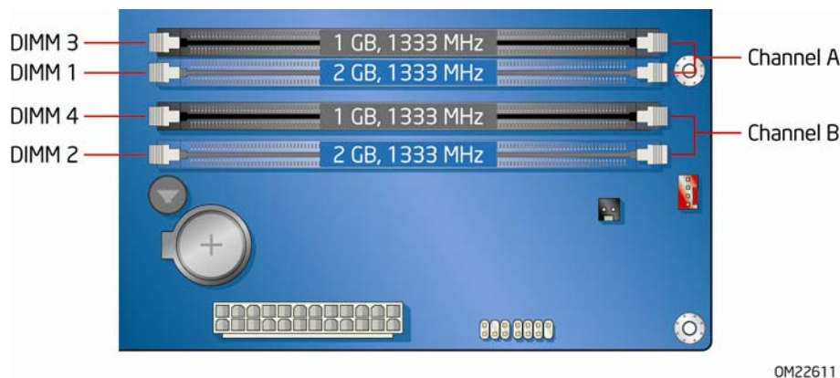
图 13. 四条 DIMM 下双通道内存配置示例
