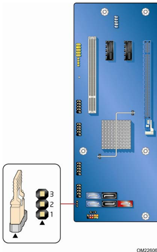
图 24. BIOS 配置跳线块位置
