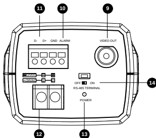
图5-2. 后面板示意图
