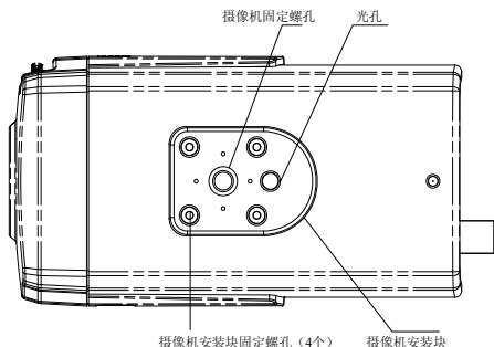
图 6-1 摄像机安装块示意图
