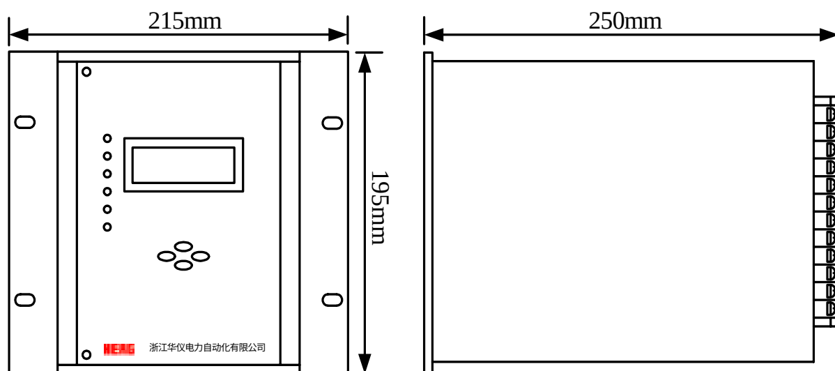
正视图
