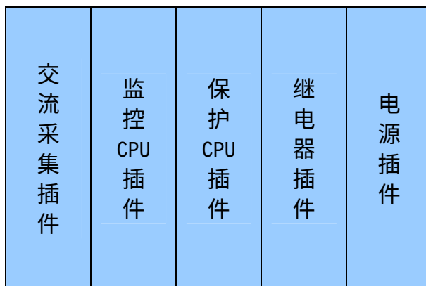
图 HYP2620 插件位置图(背视)
