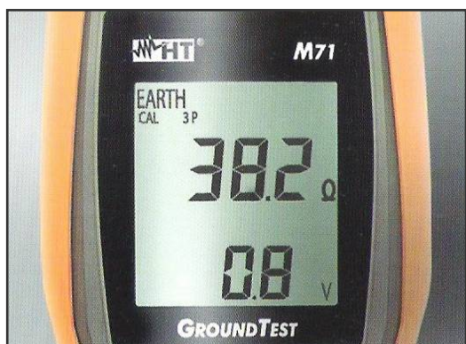
接地电阻测试 (3 线测试法) [M71]
