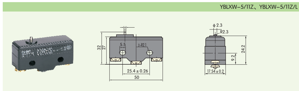
YBLXW-5/11N2、YBLXW-5/11N2/L
