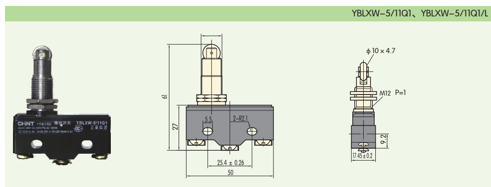
YBLXW-5/11Q2、YBLXW-5/11Q2/L
