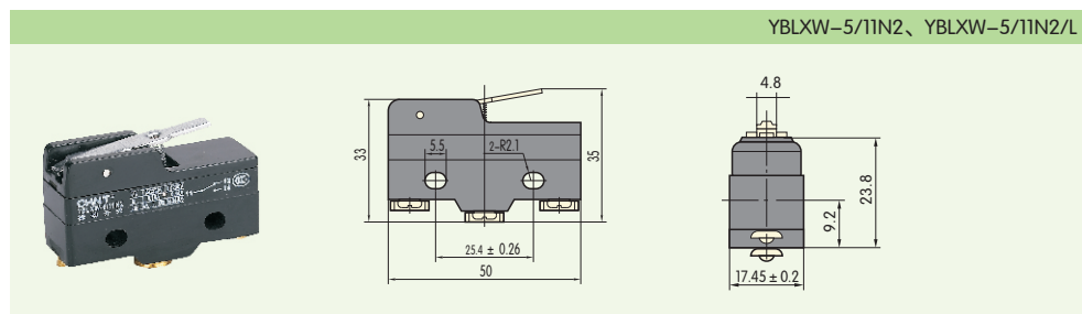
YBLXW-5/11G3、YBLXW-5/11G3/L
