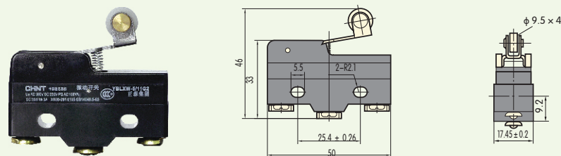
YBLXW-5/11G2、YBLXW-5/11G2/L
