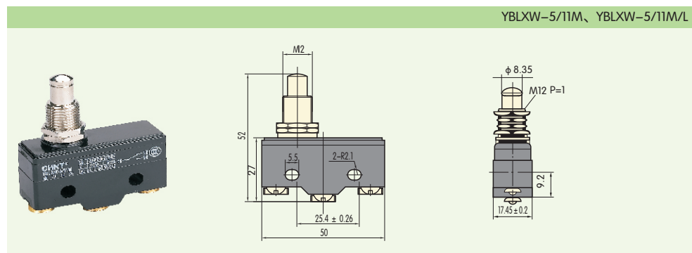
YBLXW-5/11Q1、YBLXW-5/11Q1/L
