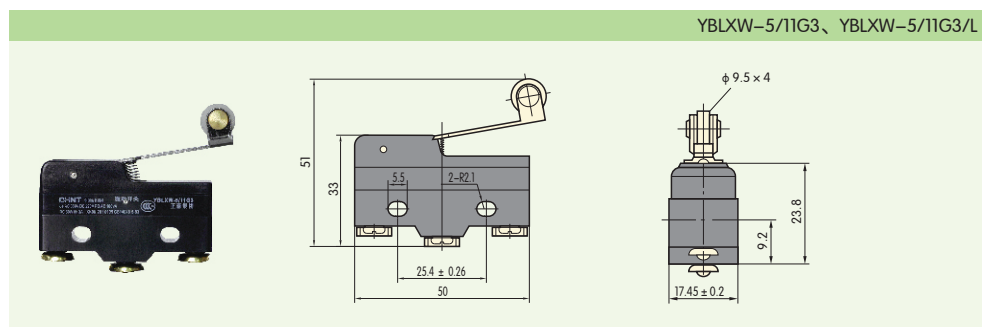
YBLXW-5/11D1、YBLXW-5/11D1/L
