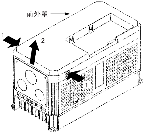
图 2. 3 取下前盖
