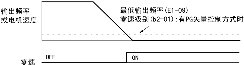
图 7.44 零速的时序图
