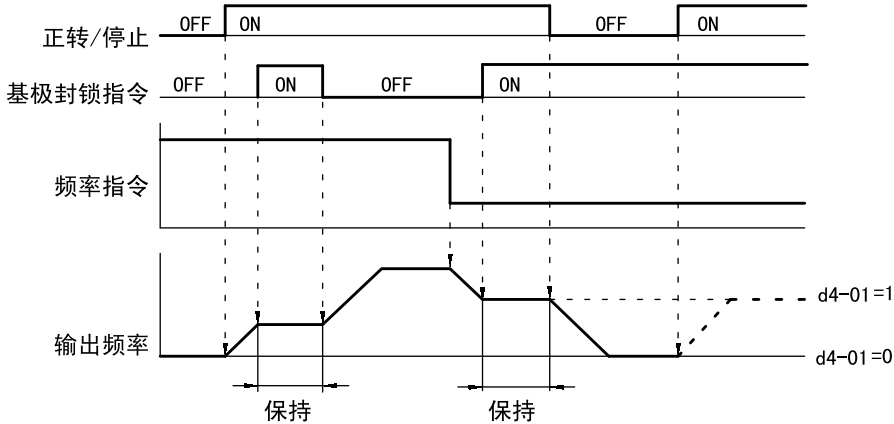
图 7.3.5 加减速停止
