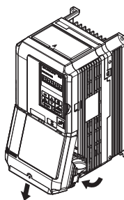
图 6 端子外罩的拆卸方法（封闭壁挂型：NEMA Type1）
