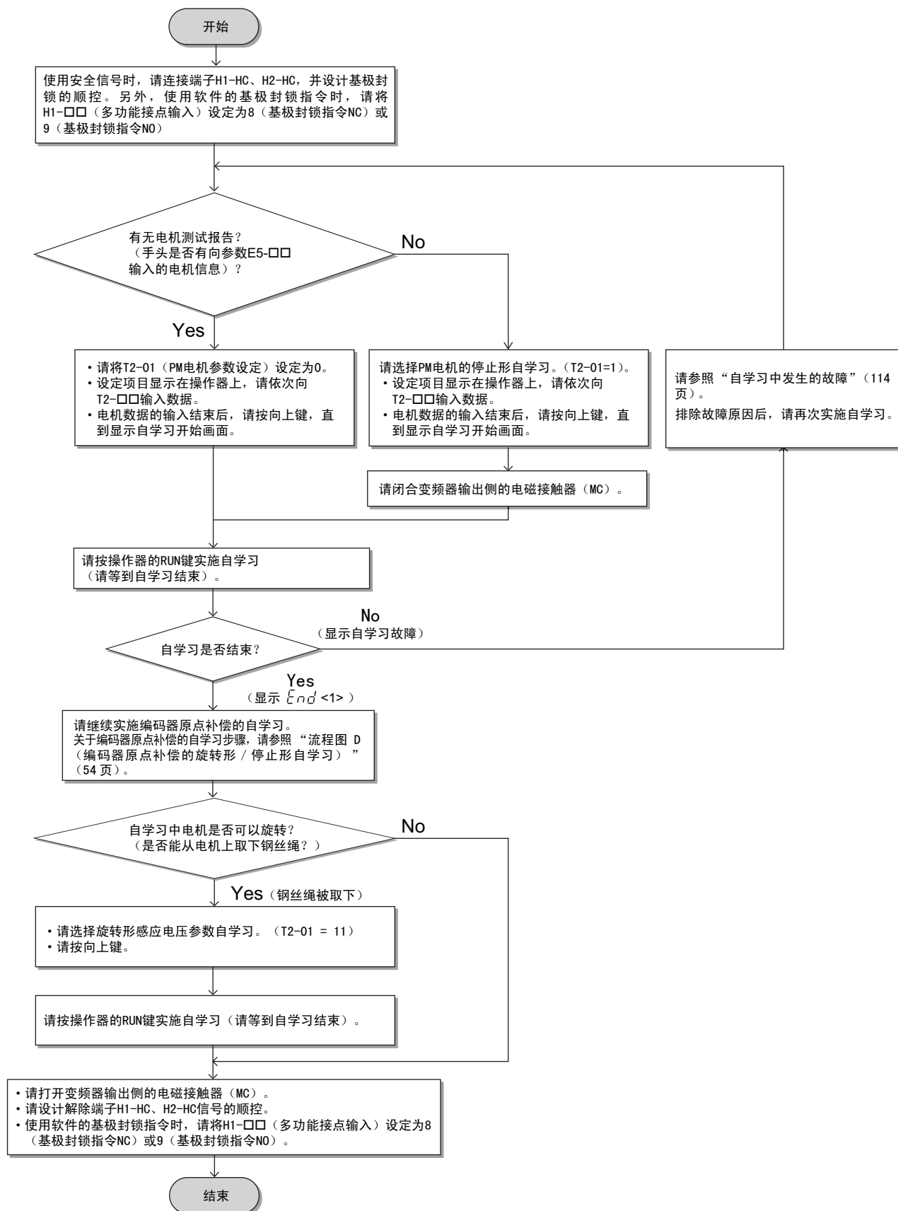
图 36 PM 电机的自学习
