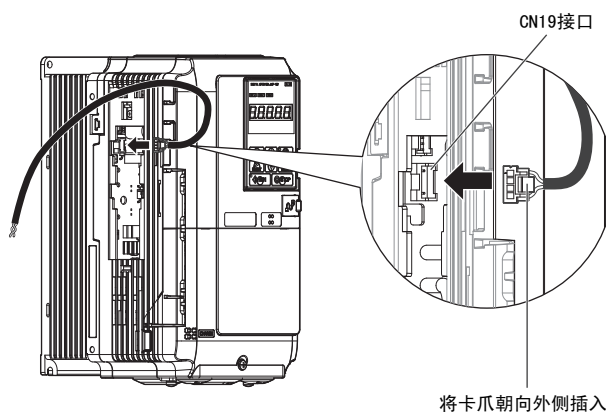
图 61 蓄电池连接用电缆的连接
