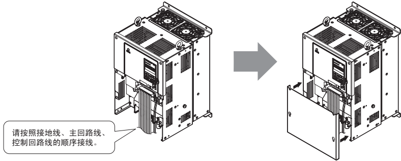
图 10 端子外罩的安装方法（柜内安装型：IP00）
