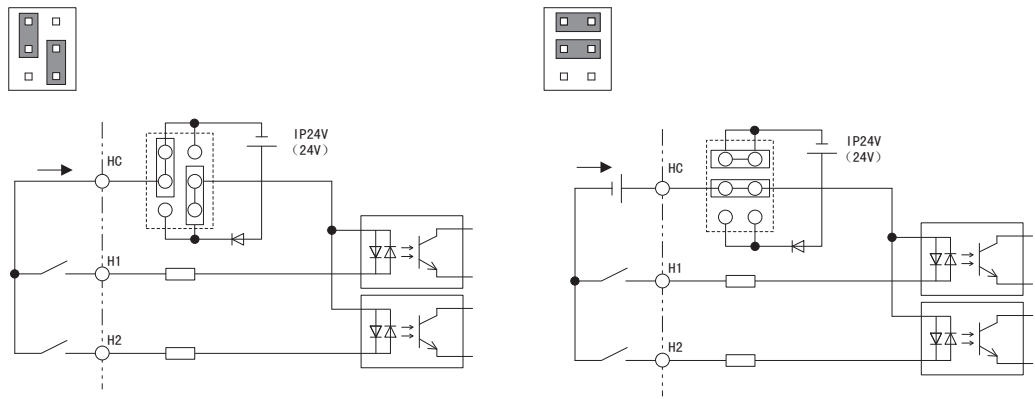
共发射极模式（0V公共点）：内部电源 共发射极模式（0V公共点）：外部电源
