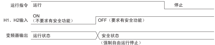
图 90 运行中将安全输入 OFF 后自由运行停止
