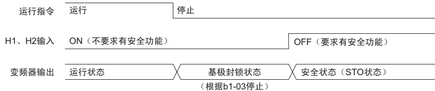
图 89 安全功能动作时的变频器状态
