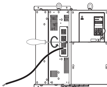
图 71 接口外罩的安装
