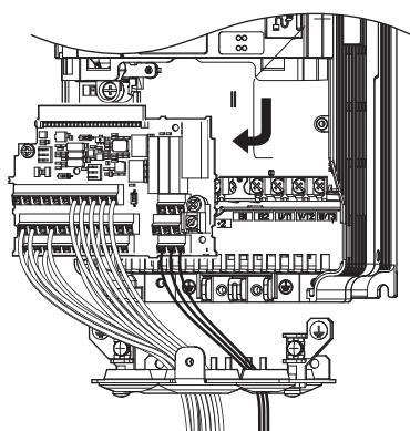
图 77 变频器的更换（端子排的拆卸）
