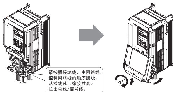
图 7 端子外罩的安装方法（封闭壁挂型：NEMA Type1）
