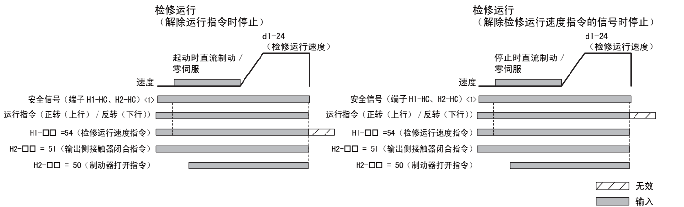
图 44 检修运行的顺序
