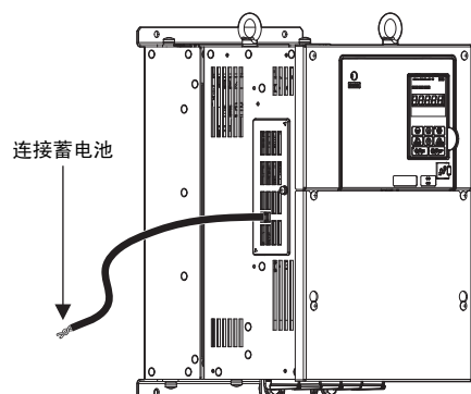
图 72 变频器蓄电池连接用电缆安装完毕的状态
