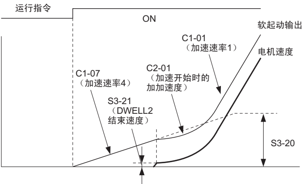
图 49 起动时的 DWELL 速度指令
