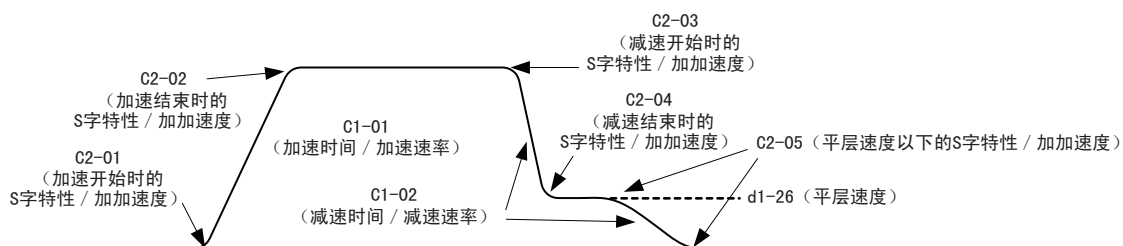
图 43 加减速时间 / 加减速速率和 S 字特性 / 加加速度
