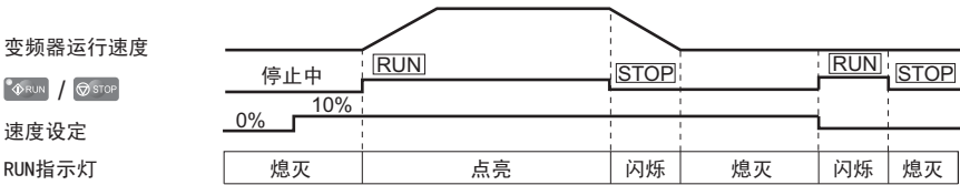
图 32 RUN 指示灯和变频器动作的关系
