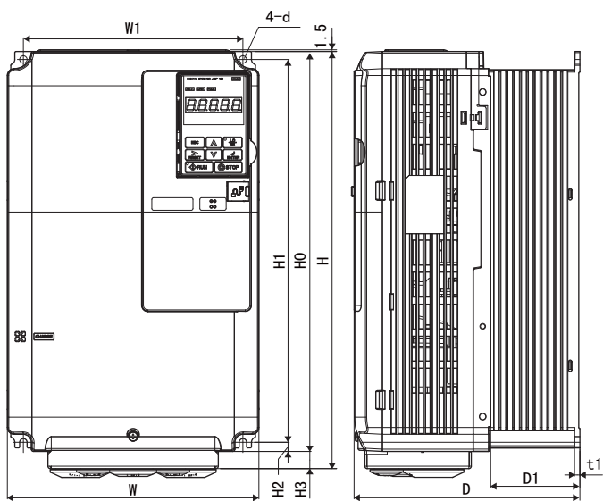
外形图2
