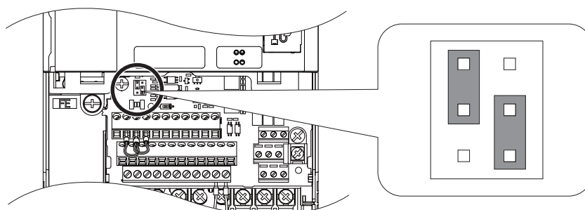
图 26 跳线 S3
