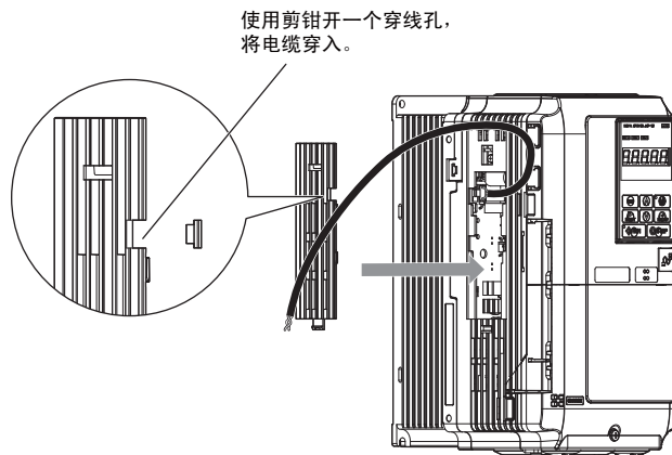
图 62 接口外罩的安装
