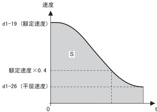
图 50 一般运行时的速度
