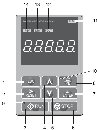
图 30 操作器各部分的名称与功能
