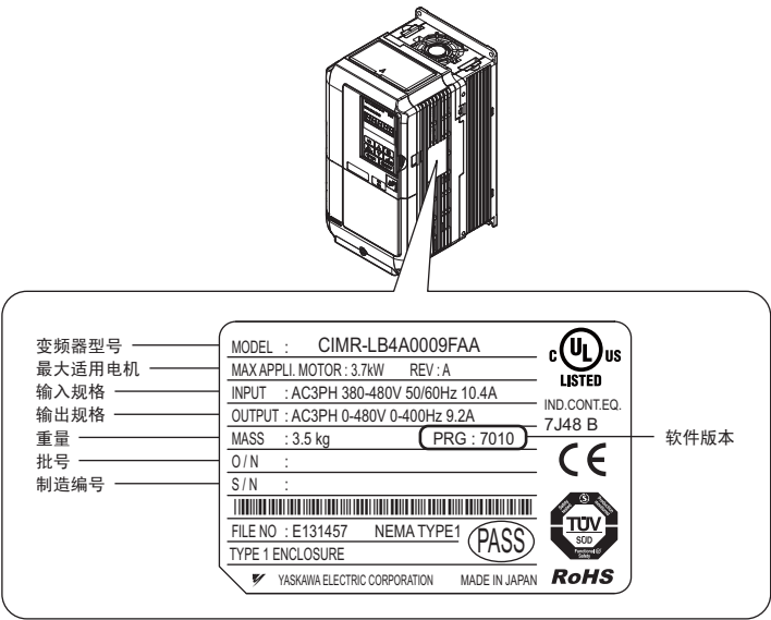
图 1 变频器的铭牌
