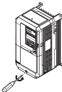
图 5 端子外罩的拆卸方法（封闭壁挂型：NEMA Type1）
