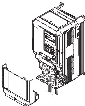
图 75 变频器的更换（端子外罩的拆卸）
