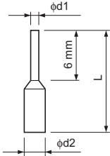
图 21 棒端子的外形尺寸图
