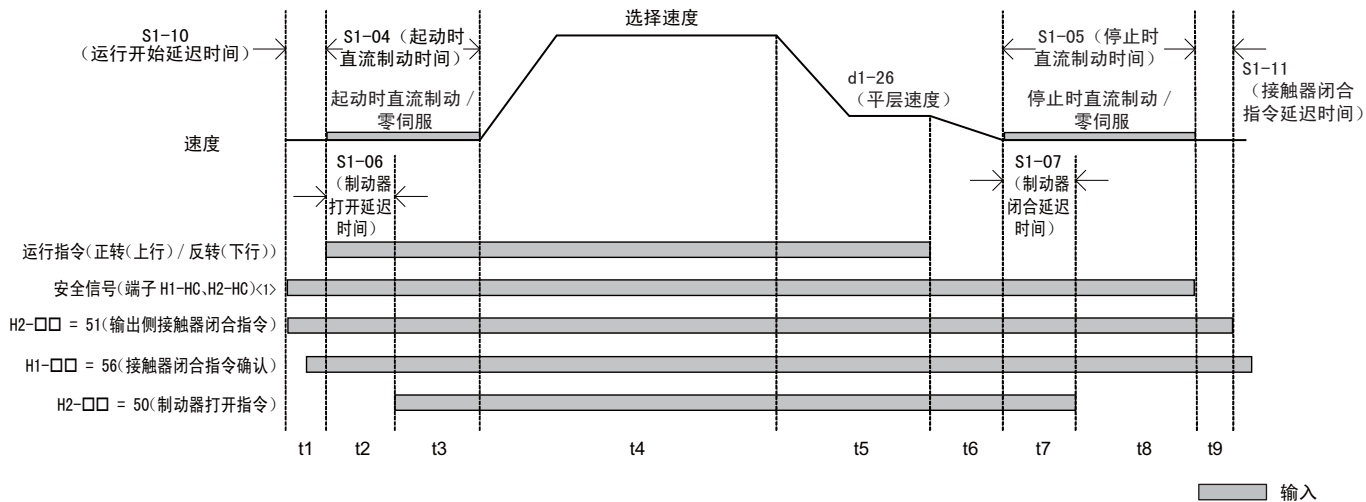
图 45 起动时无转矩补偿的制动器顺控的时序图
