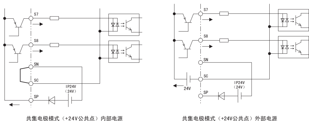
图 25 共集电极模式（+24V 公共点）
