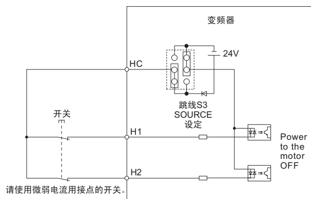
图 93 安全输入的连接示例（双工化）
