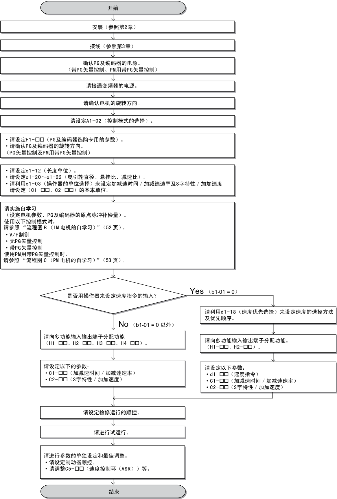
图 34 从安装、接线到电机及电梯调整的基本步骤
