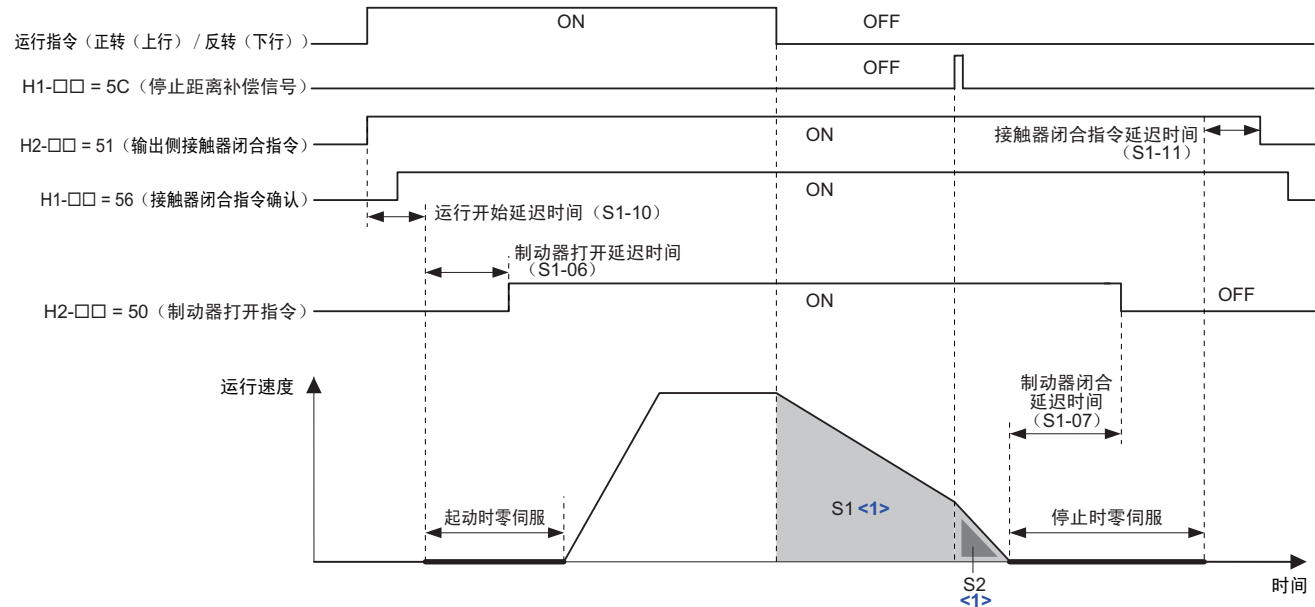
图 52 直接平层的运行顺控示例
