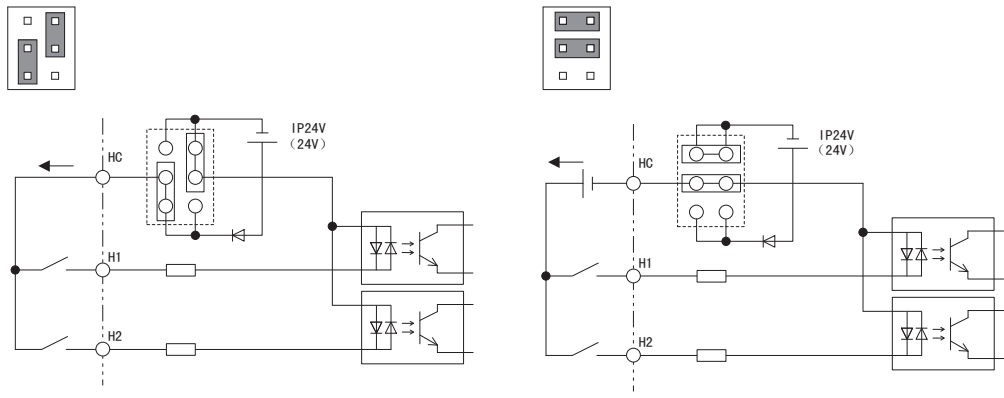
共集电极模式（+24V公共点）内部电源 共集电极模式（+24V公共点）外部电源
