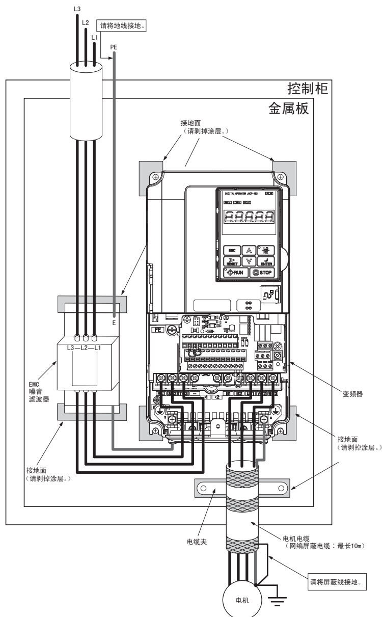
图 84 EMC 噪音滤波器和变频器的安装方法 (三相 200V/400V 级)
