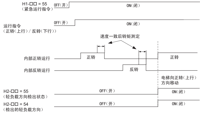
图 73 轻负载方向检出的时序图（检出正转方向时）
