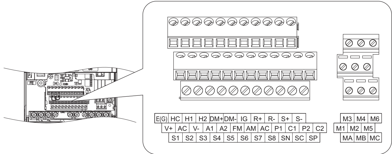
图 20 带参数备份功能的拆装式端子排的排列 (C1MR-LB□A□□□□□□□□)
