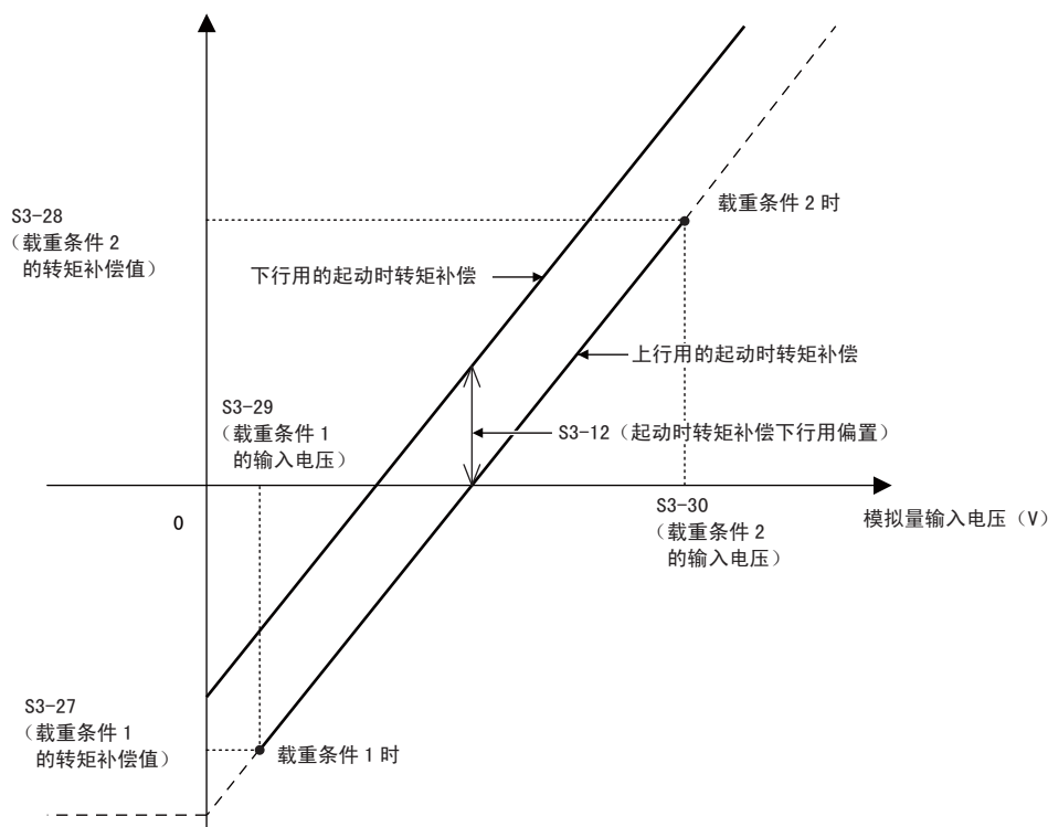
图 47 上行用起动时转矩补偿与下行用起动时转矩补偿
