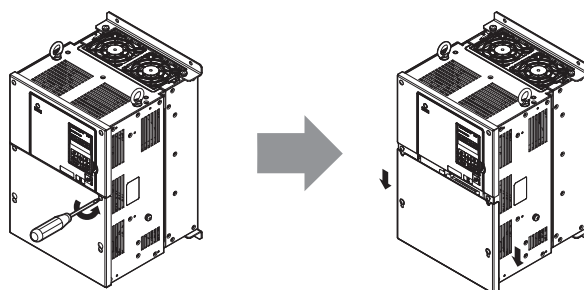
图 8 端子外罩的拆卸方法（柜内安装型：IP00）
