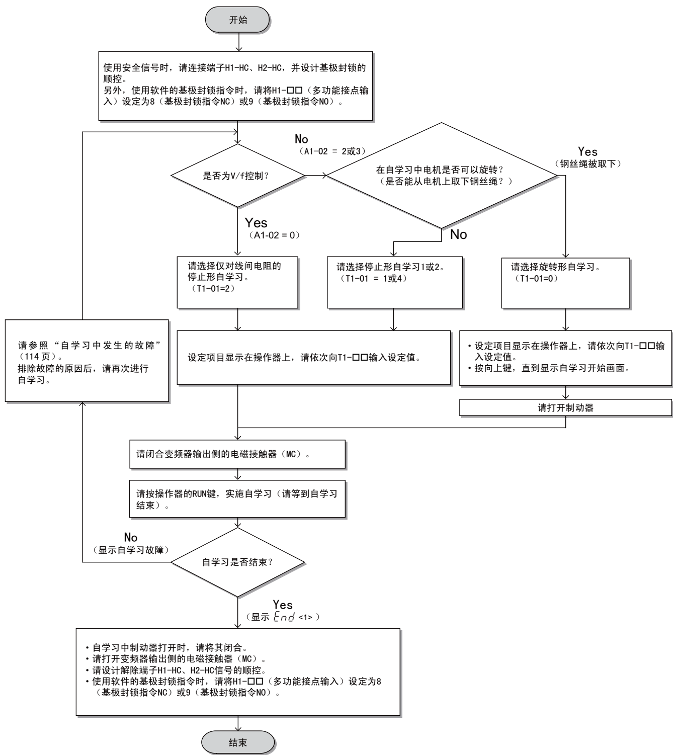
图 35 IM 电机的自学习
