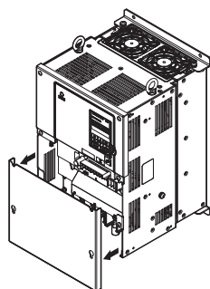
图 9 端子外罩的拆卸方法（柜内安装型：IP00）
