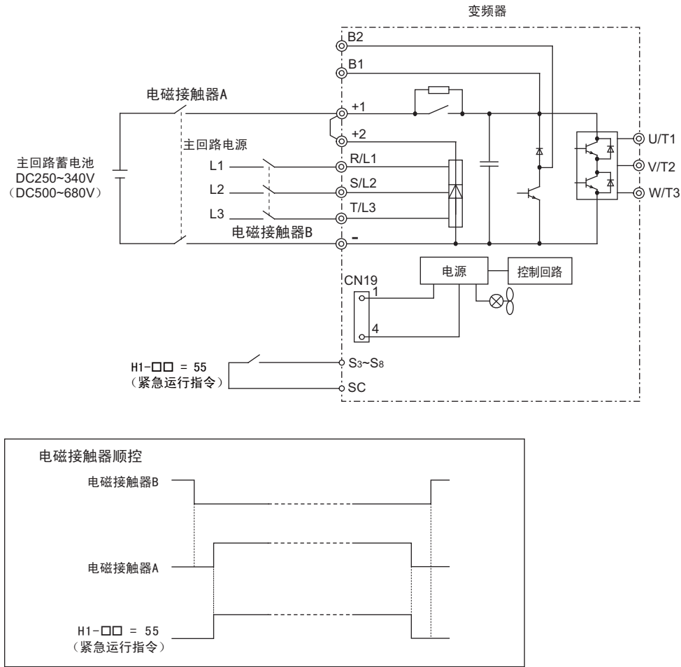
图 59 仅主电源侧使用蓄电池，蓄电池电压在 DC250V（200V 级）/DC500V（400V 级）以上时
