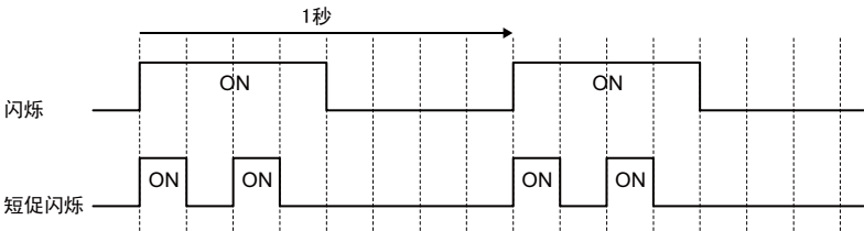
图 31 关于 RUN 指示灯的闪烁状态
