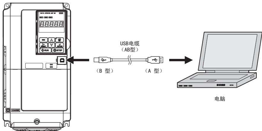
图 29 与电脑的连接（USB）
