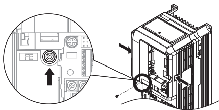
图 13 前外罩的拆卸
