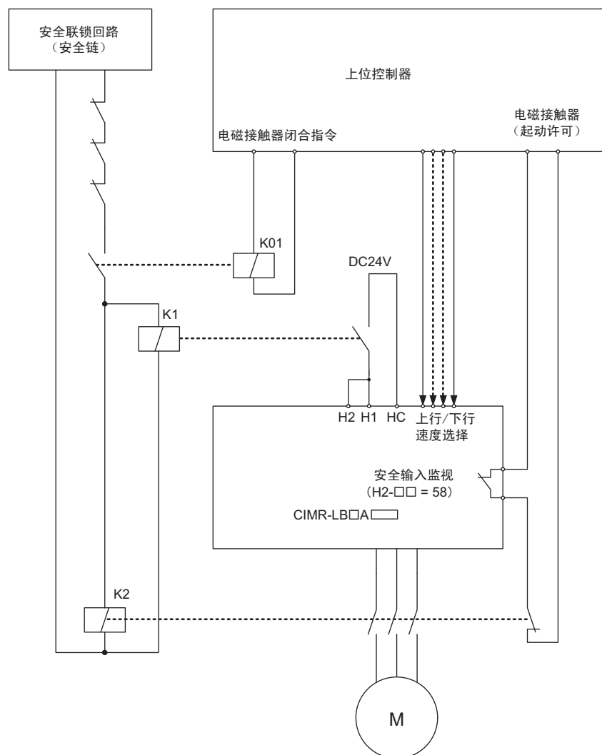
图 95 符合标准的接线示例（1 个变频器输出侧电磁接触器）
