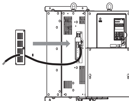
图 69 接口外罩的安装
