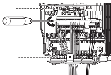
图 76 变频器的更换（拧松固定螺丝）
