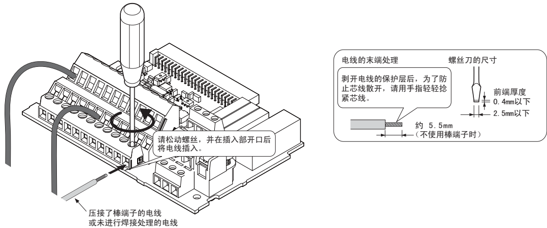
图 22 控制回路的接线步骤
