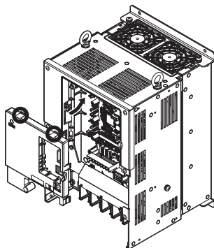
图 14 安装前外罩（2A0085 ~ 2A0415、4A0045 ~ 4A0216）
