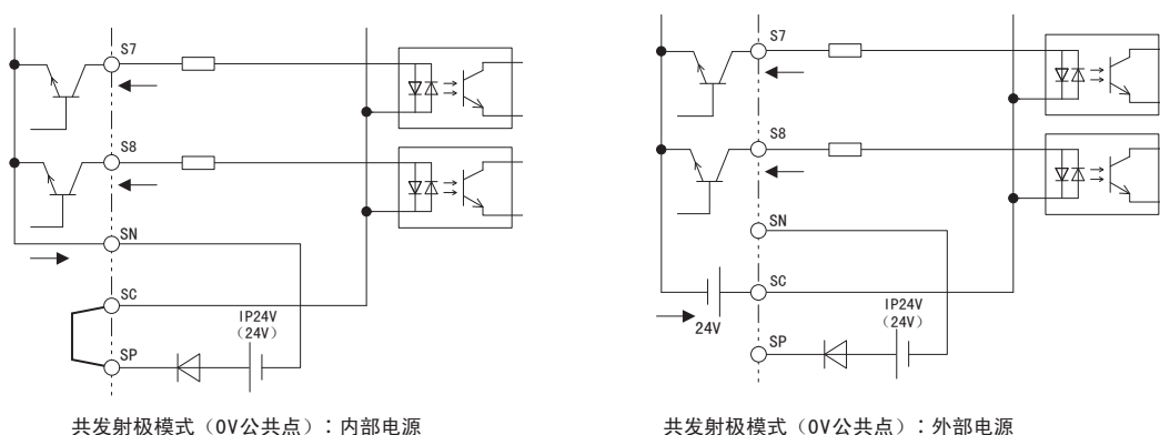
图 24 共发射极模式（0V 公共点）
