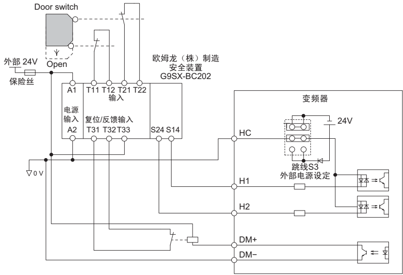
图 94 安全功能的连接示例
