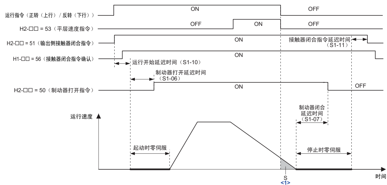
图 53 平层距离控制的运行顺控示例
