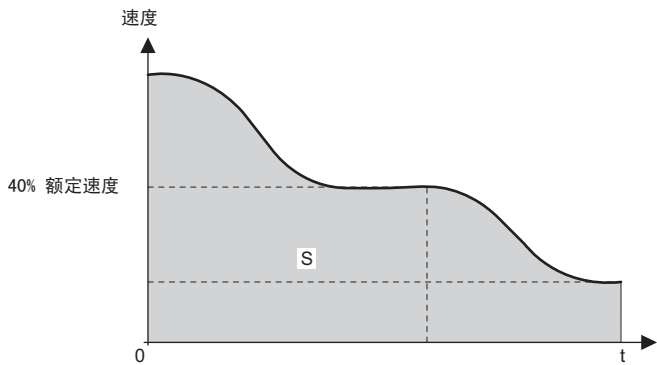
图 51 短楼层功能
