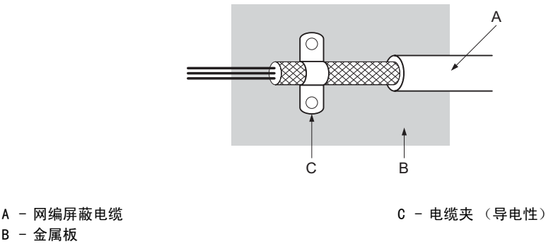
图 83 电缆的接地方法
