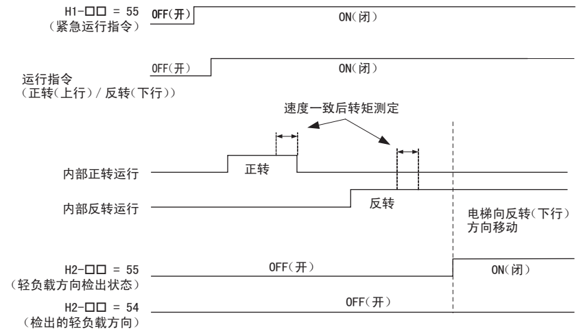
图 74 轻负载方向检出的时序图（检出反转方向时）
