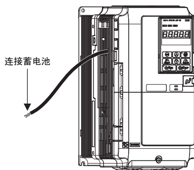
图 64 变频器蓄电池连接用电缆安装完毕的状态
