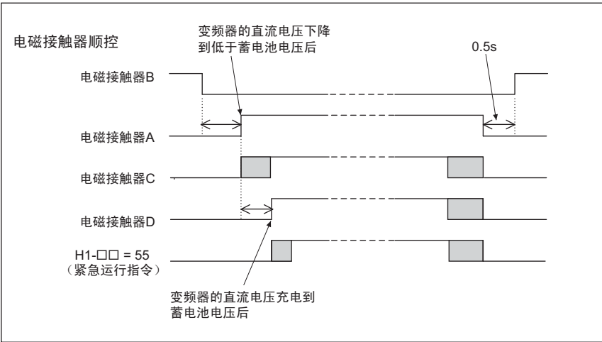
图 56 主电源、控制电源均使用蓄电池，主电源侧的蓄电池电压在 DC250V（200V 级）以下时 (CIMR-LB2A0215 ~ 0415、CIMR-LB4A0180 ~ 0216)
