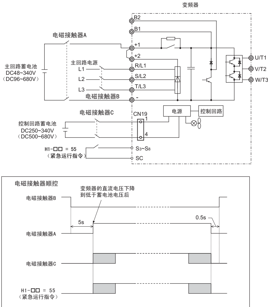
图 55 主电源、控制电源均使用蓄电池，主电源侧的蓄电池电压在 DC250V（200V 级）/DC500V（400V 级）以下时（C1MR-LB2A0009 ~ 0180、C1MR-LB4A0018 ~ 0150）
