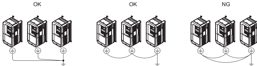
图 17 多台变频器的接线
