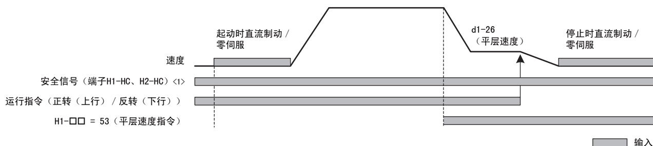
图 42 平层速度指令优先时, 不选择 H1-□□ = 50 (额定速度指令) 时的速度指令
