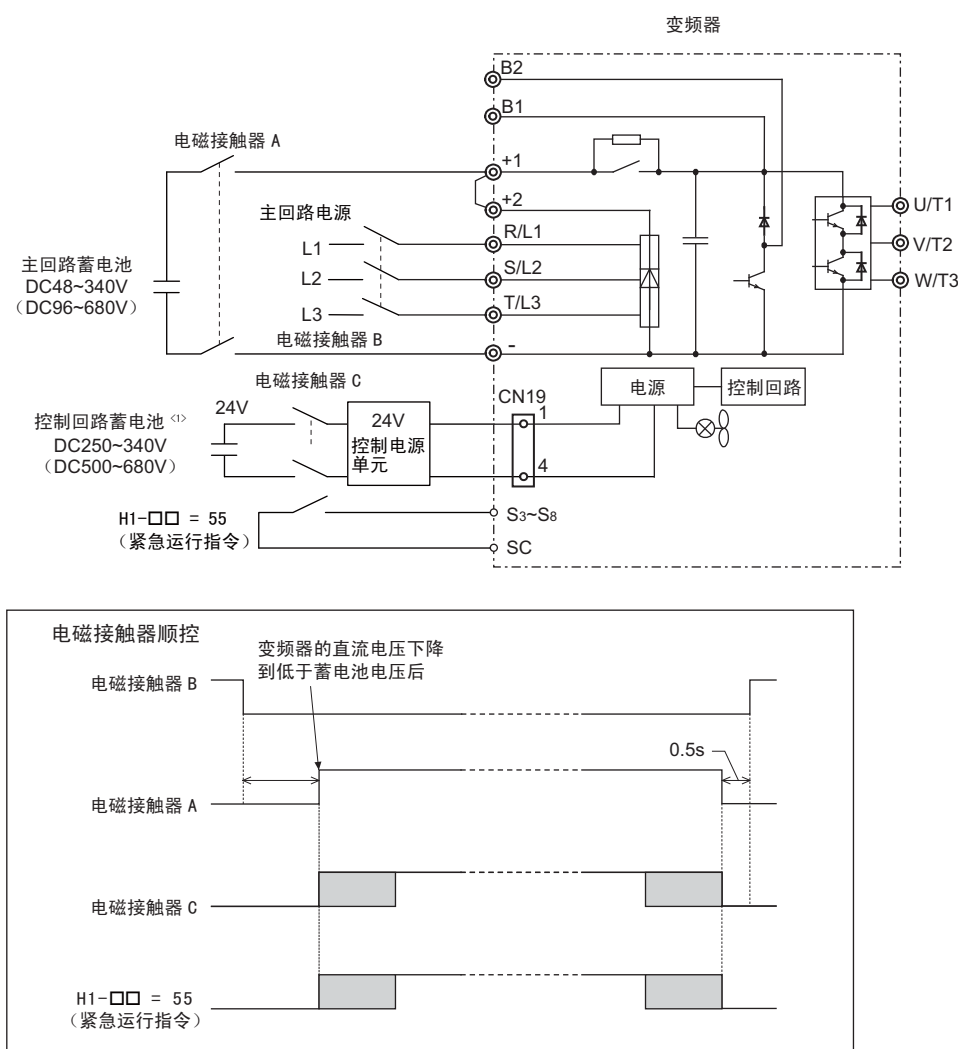
图 57 主电源侧使用蓄电池，控制电源侧使用 24V 控制电源单元时 (C1MR-LB2A0009 ~ 0180、C1MR-LB4A0018 ~ 0150)
