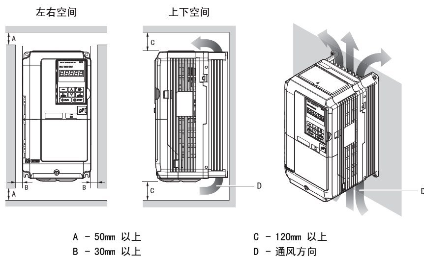
图 3 变频器的安装空间（单机）
