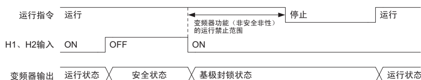
图 92 从安全状态（STO 状态）返回 (运行中 H1、H2 输入为 OFF，进入安全状态时)
