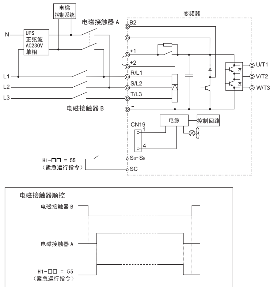
图 54 使用单相 230V 的 UPS 时
