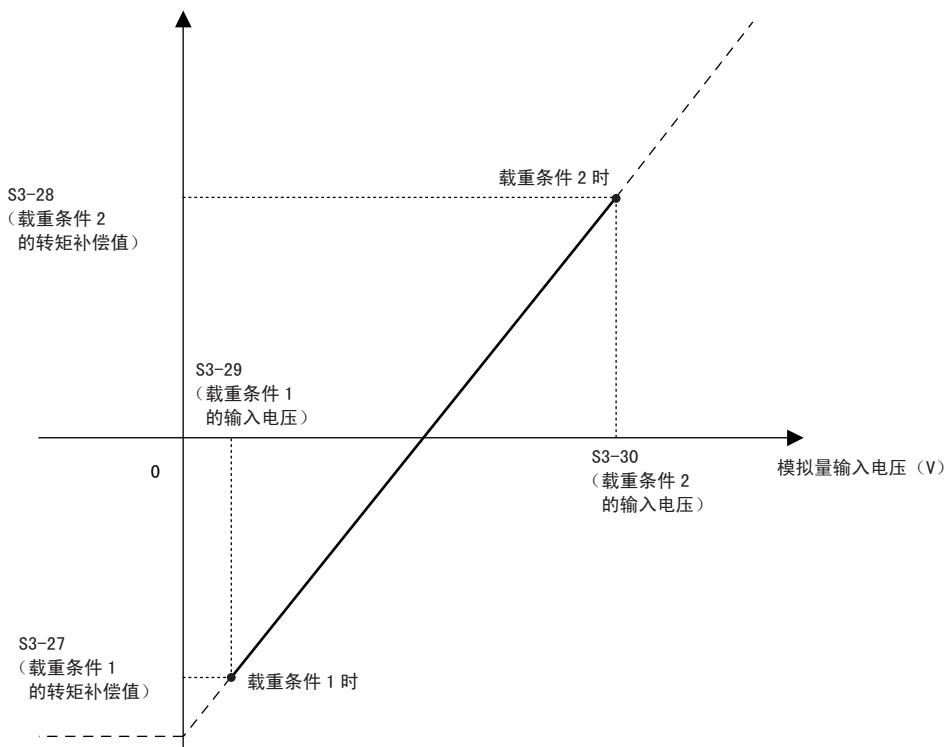
图 46 起动时转矩补偿
