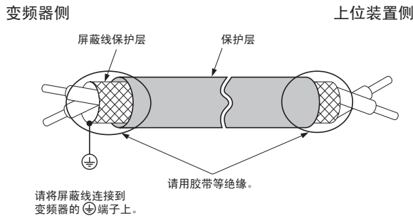
图 23 屏蔽线的线头处理
