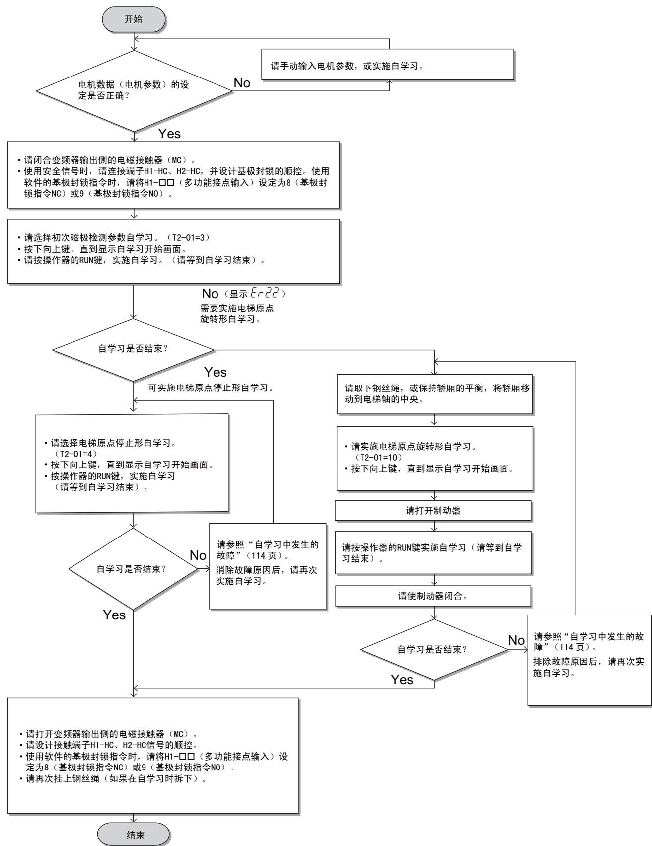
图 37 编码器原点补偿的旋转形 / 停止形自学习
