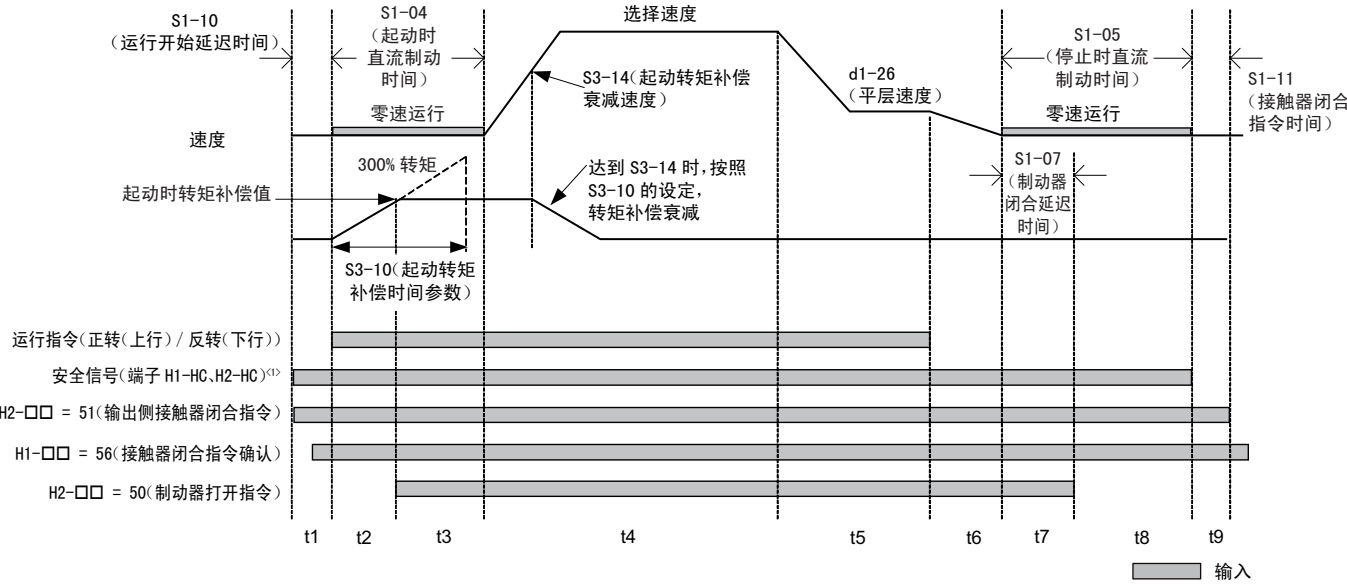
图 48 启动时有转矩补偿的制动器顺控的时序图
