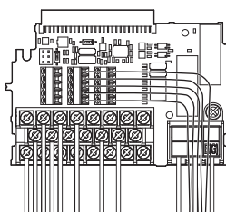
图 78 变频器的更换 (已拆下的拆装式端子排)
