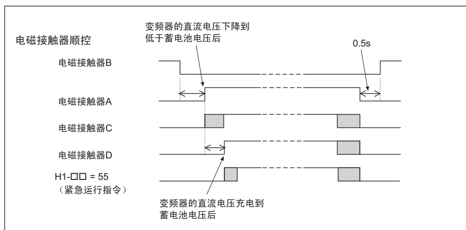
图 58 主电源侧使用蓄电池，控制电源侧使用 24V 控制电源单元时 (C1MR-LB2A0215 ~ 0415、C1MR-LB4A0180 ~ 0216)
