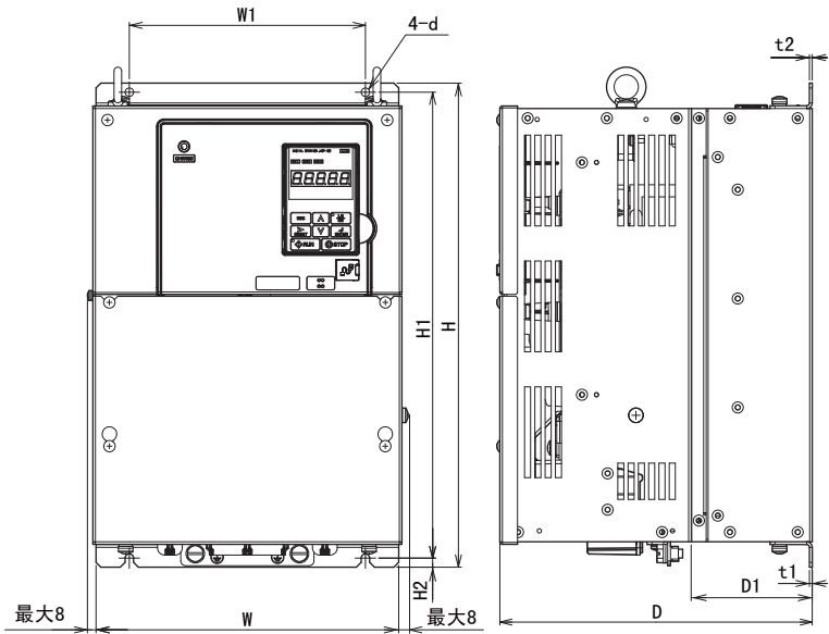
外形图1
