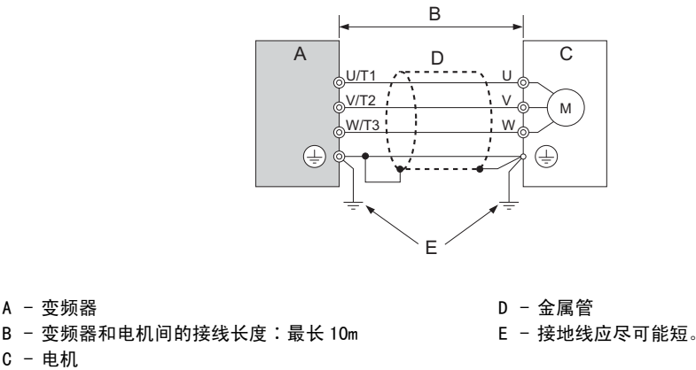
图 82 安装方法
