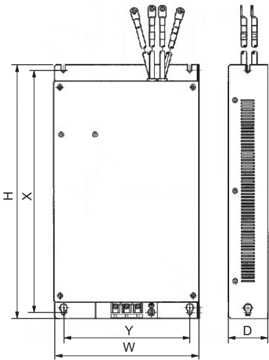
外形图1
