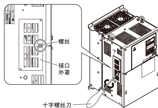
图 65 接口外罩的拆卸
