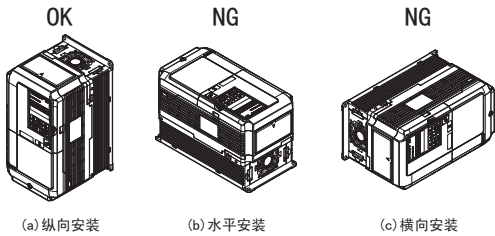
图 2 安装方向
