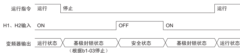
图 91 从安全状态（STO 状态）返回
