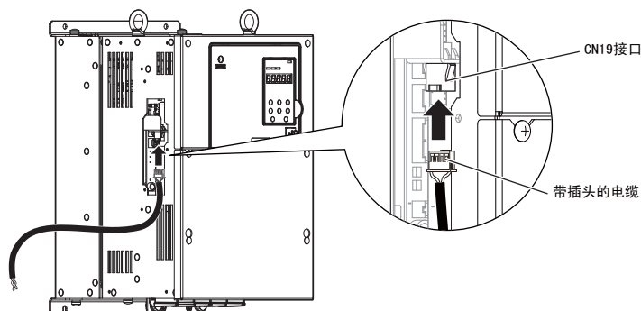
图 68 蓄电池连接用电缆的连接
