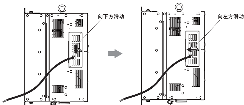
图 70 接口外罩的滑动方向
