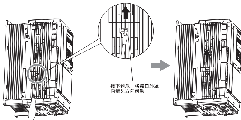
图 60 接口外罩的拆卸
