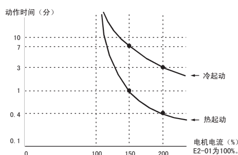
图 87 由输出频率和负载决定的电机过载保护时间
