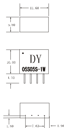
DY XXSXXS-1W 封装模式
