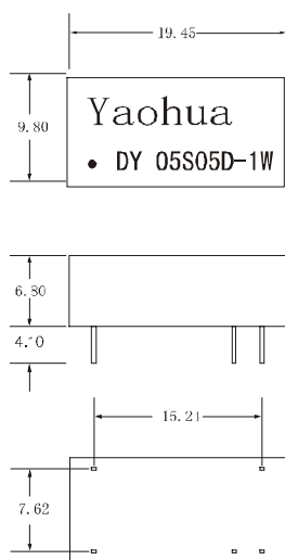
DY XXSXXD-1W封装模式
