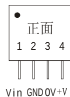
(侧视)
