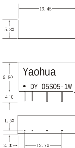
DY XXSXX-1W 封装模式
