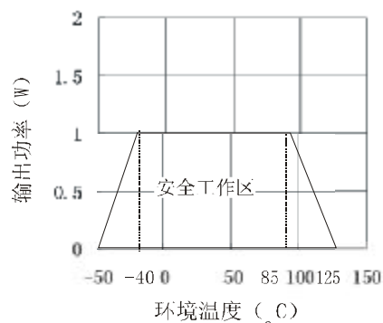
温度特性:
