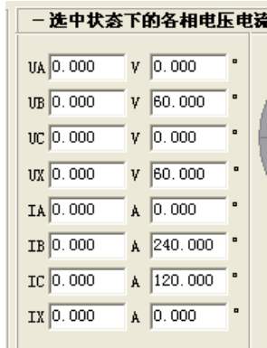
故障中
