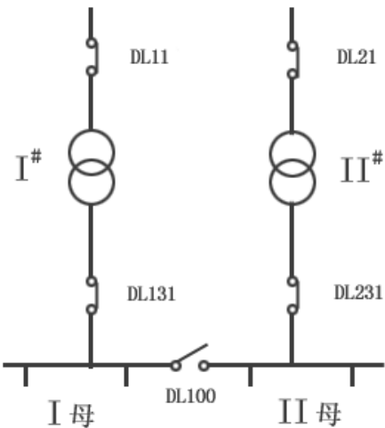
明备用
