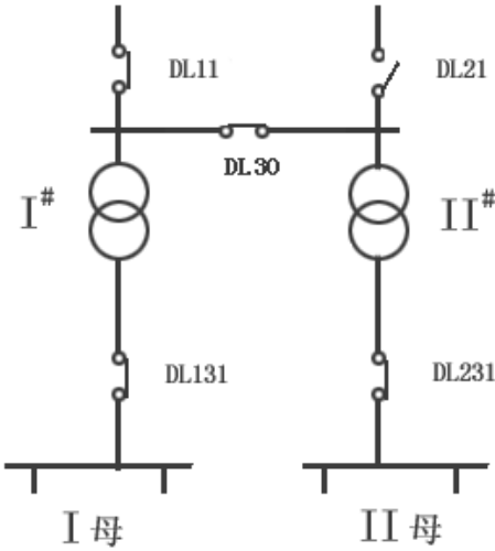
暗备用
