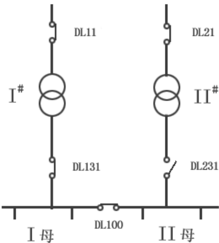
暗备用
