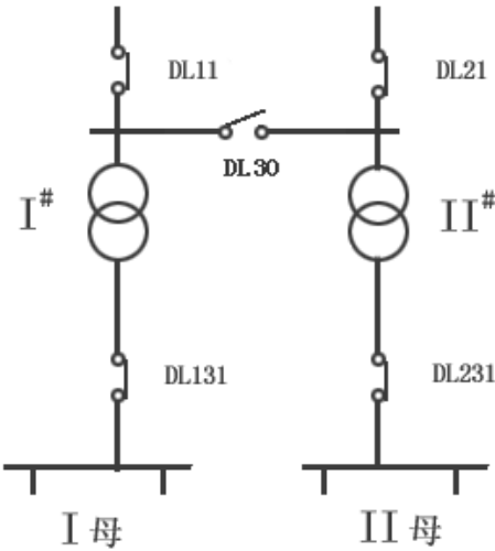
明备用
