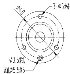
光准直器尺寸图
