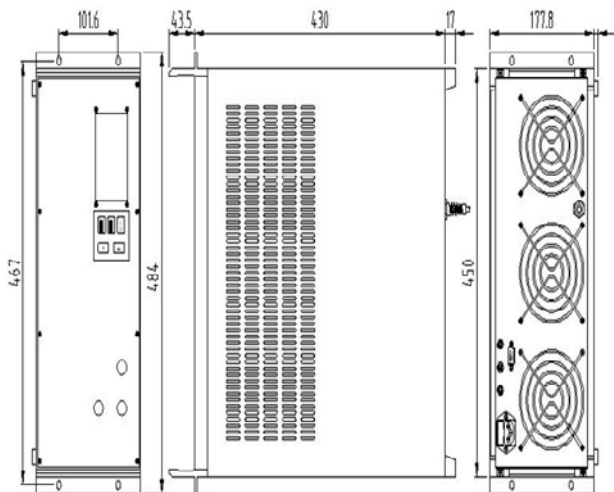
激光模块尺寸图
