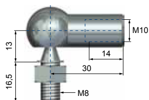
2-M10 Winkelgelenk • Angle joint Joint à angle • Snodo angolare Charnela articulada
