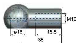
Kugelpfanne • Ball joint housing Coussinet sphérique Cuscinetto sferico Cojinete esférico
