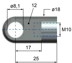
1-M10 Gelenkauge • Male rod clevis Tête de chape (male) Attacco a cerniera maschio Charnela macho
