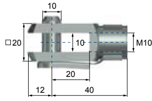
3-M10 Gabelkopf • Female rod clevis Embout à rotule (femelle) Forcella femmina Charnela hembra
