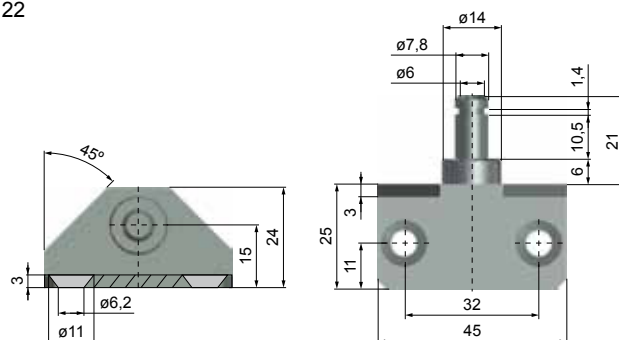
Kugelpfanne • Ball joint housing Coussinet sphérique Cuscinetto sferico Cojinete esférico
