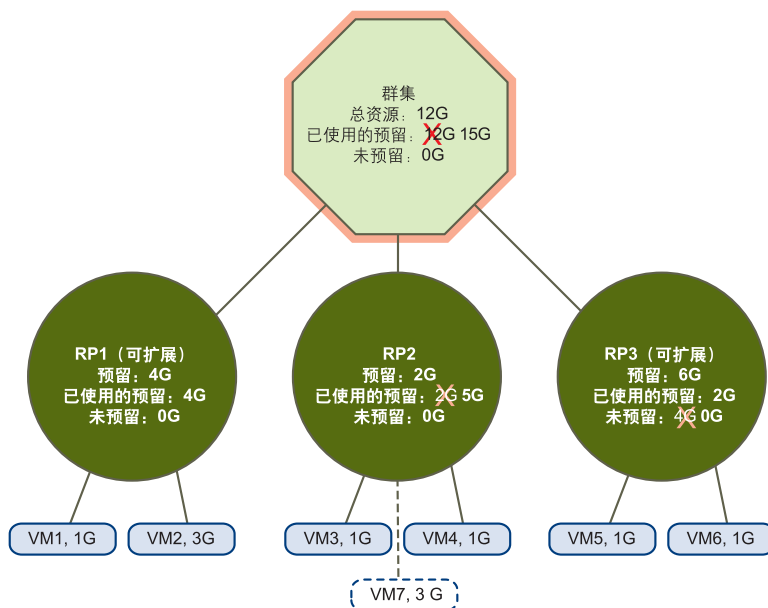
图 4-13. 红色群集
