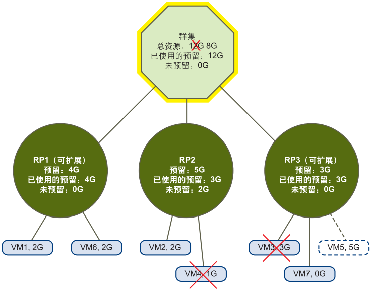
图 4-12. 黄色群集
