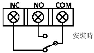
內部接線圖
