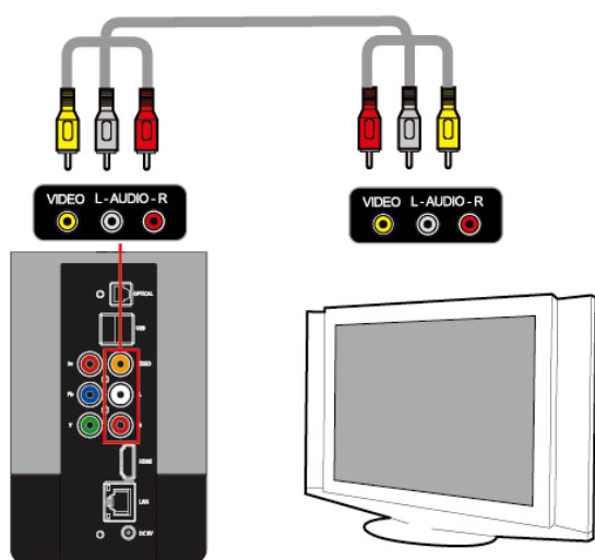
一般TV输出连接
