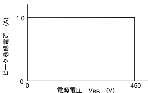
図 1: T_j = 135 \text{ }^\circ\text{C} の安全動作領域
