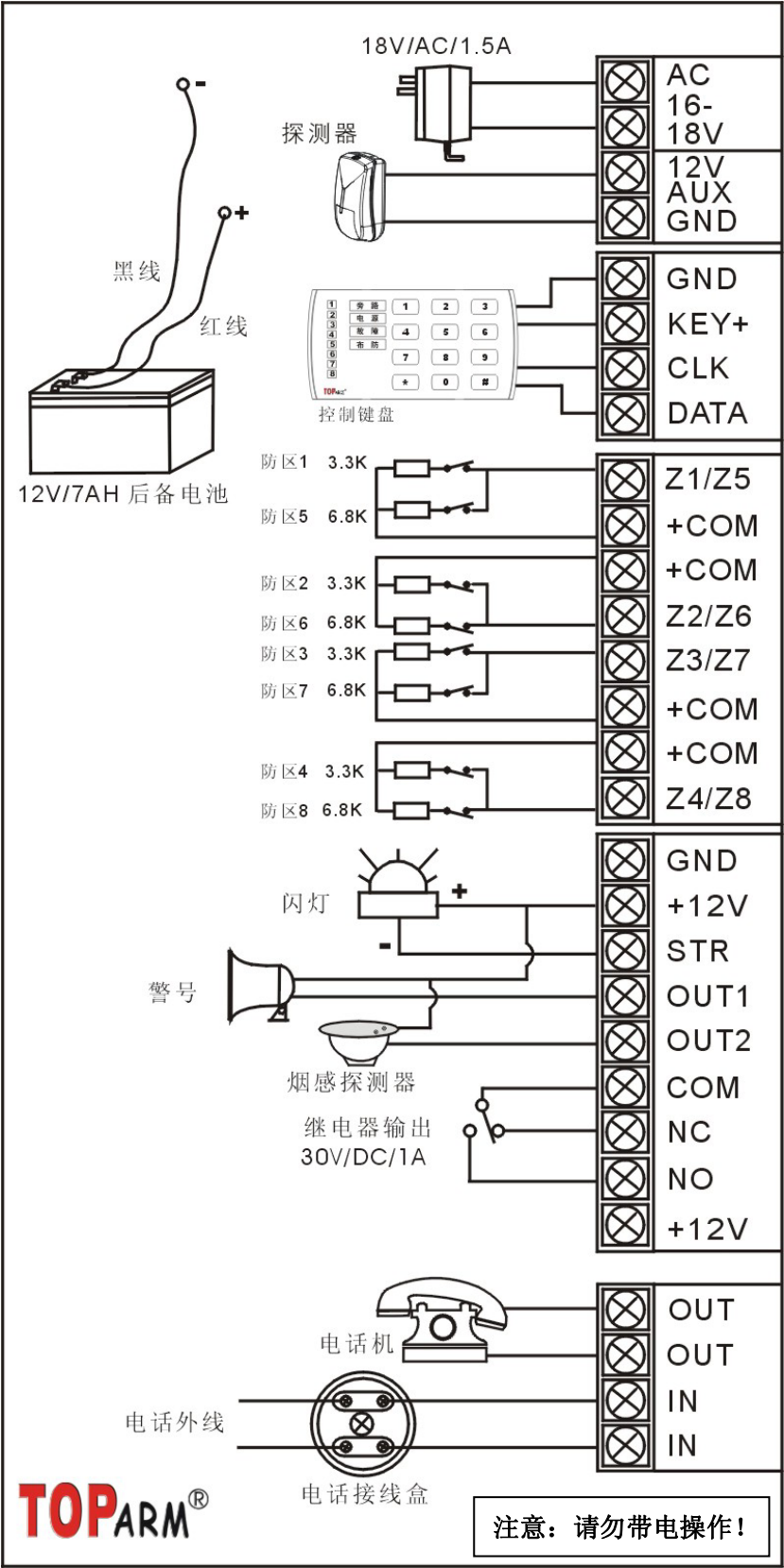
TP428 接线图
