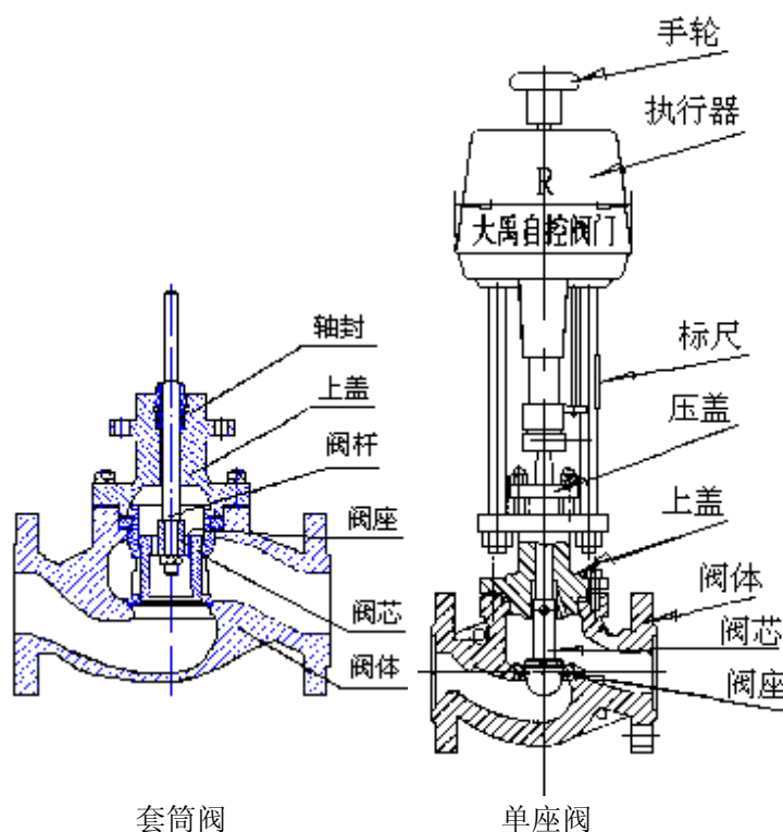
图 1 调节阀结构图
