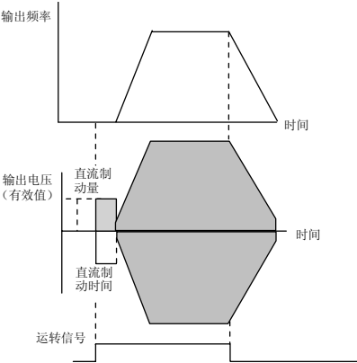
图6-8 启动方式1说明
