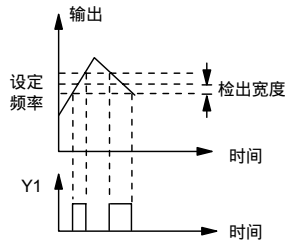
图6-22 频率到达信号输出示意图
