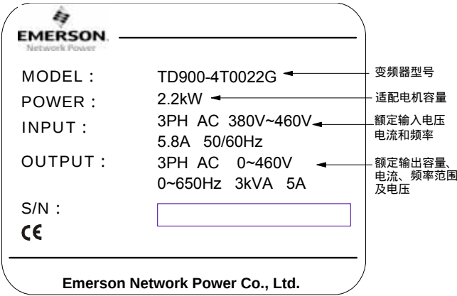
图2-1 变频器铭牌
