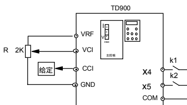
图4-4 操作配线图
