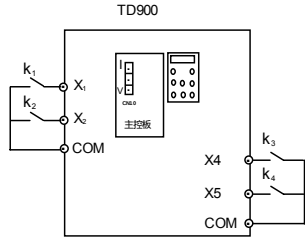
图4-3 多段速度运行接线图
