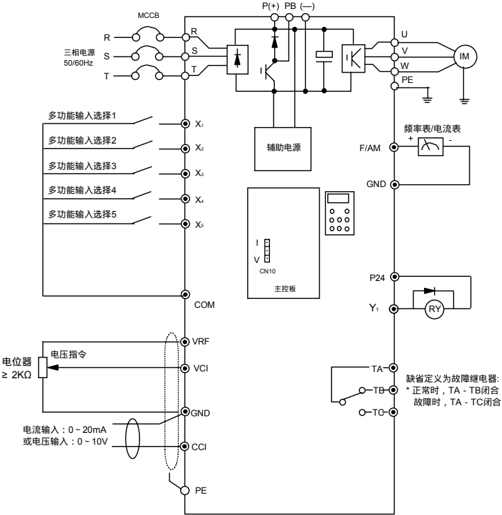
图3-6 基本配线图
