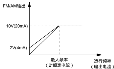
图6-25 FM/AM输出示意图（校正系数为100%）
