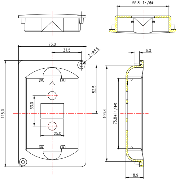
键盘安装座的外形与安装尺寸
