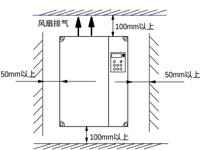
图3-3 安装的间隔距离
