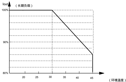
图2-2 降额示意图
