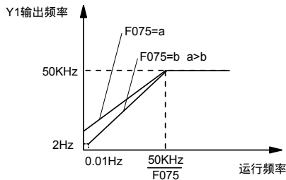
图6-24 数字频率输出示意图
