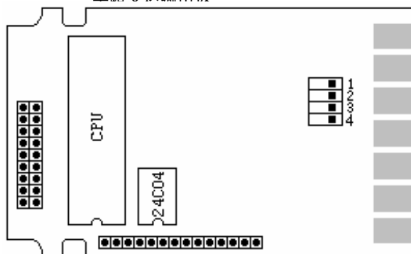
单路变送输出板
