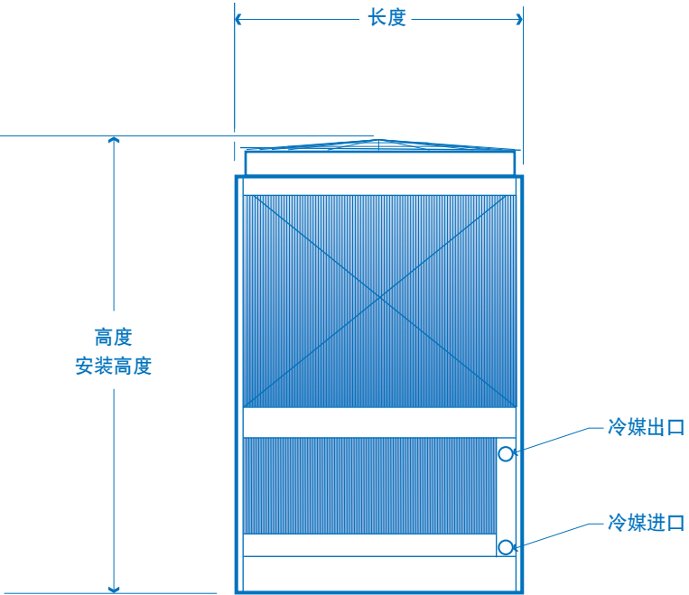
讲风门面立面图
