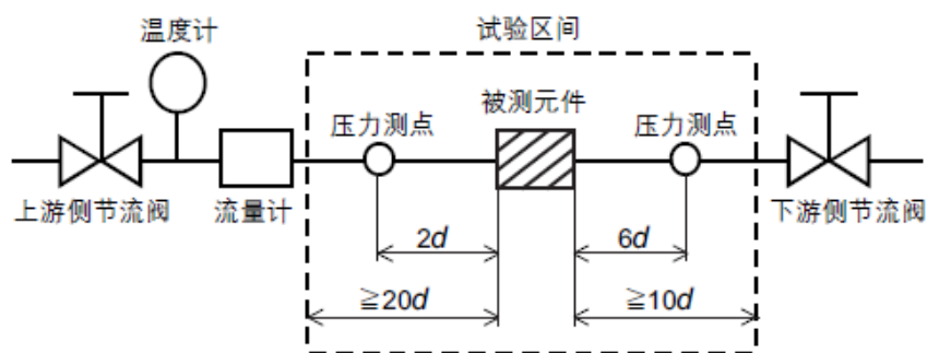
图5.依据IEC60534-2-3、JIS B 2005的试验回路
