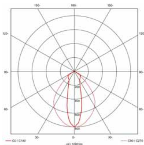
配光曲线 ( LDC ):
