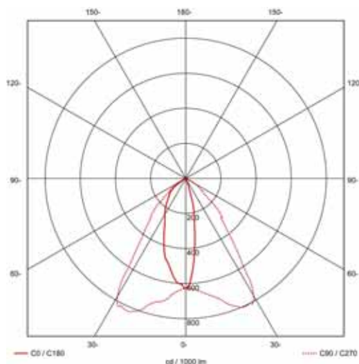
配光曲线 (LDC)
