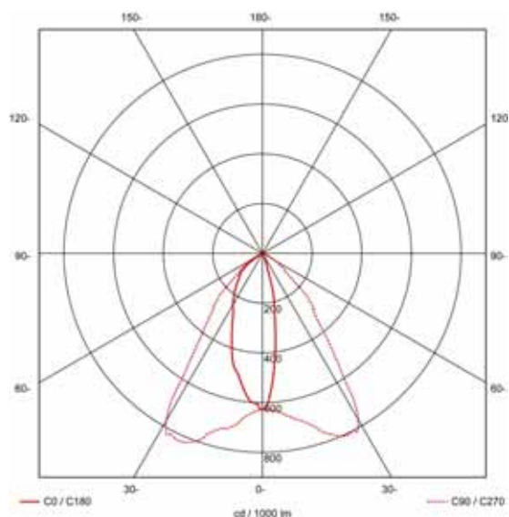
配光曲线 (LDC)
