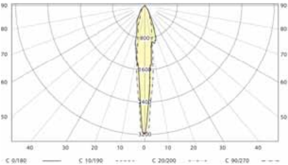
配光曲线 ( LDC ) :
