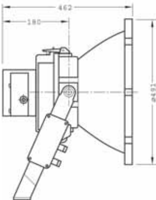
尺寸图 ( Dimension Drawing ) :
