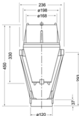
尺寸图 ( Dimension Drawing ) :
