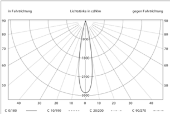
配光曲线 (LDC)
