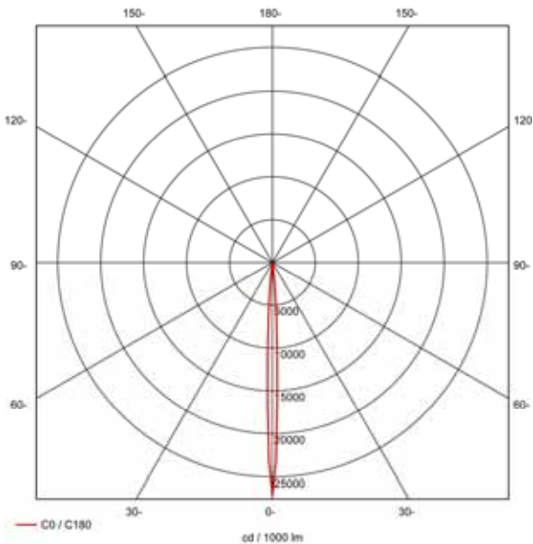
配光曲线 ( LDC )
