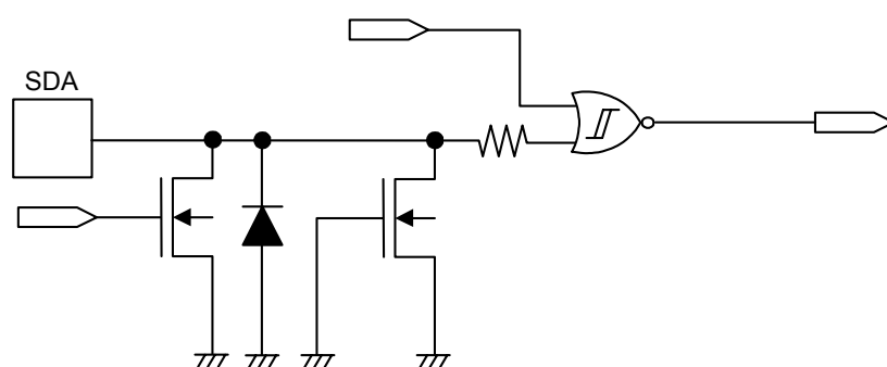
图23 SDA端子
