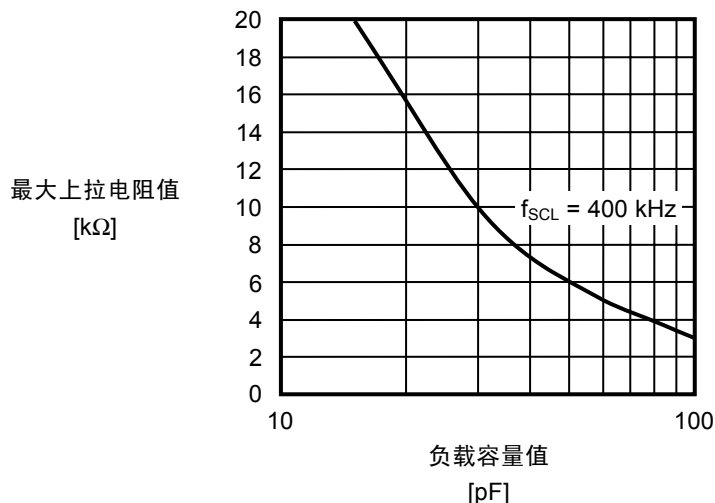
图9 输出负载
