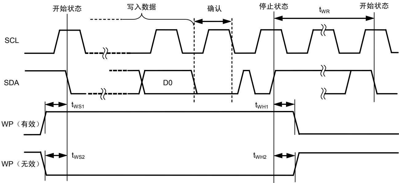
图8 写入周期定时
