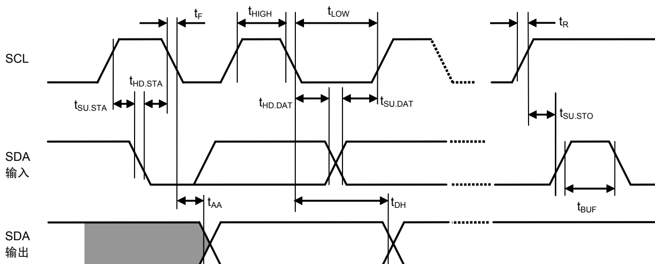
图7 总线定时
