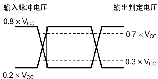
图6 AC测量输入、输出波形
