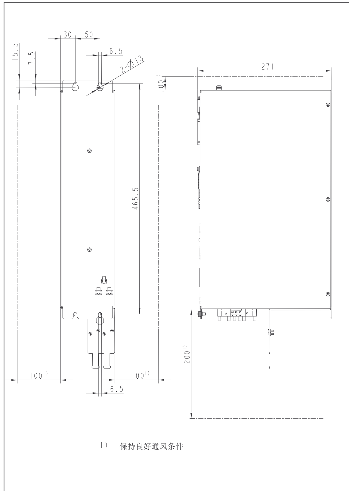
图2-1 安装尺寸
