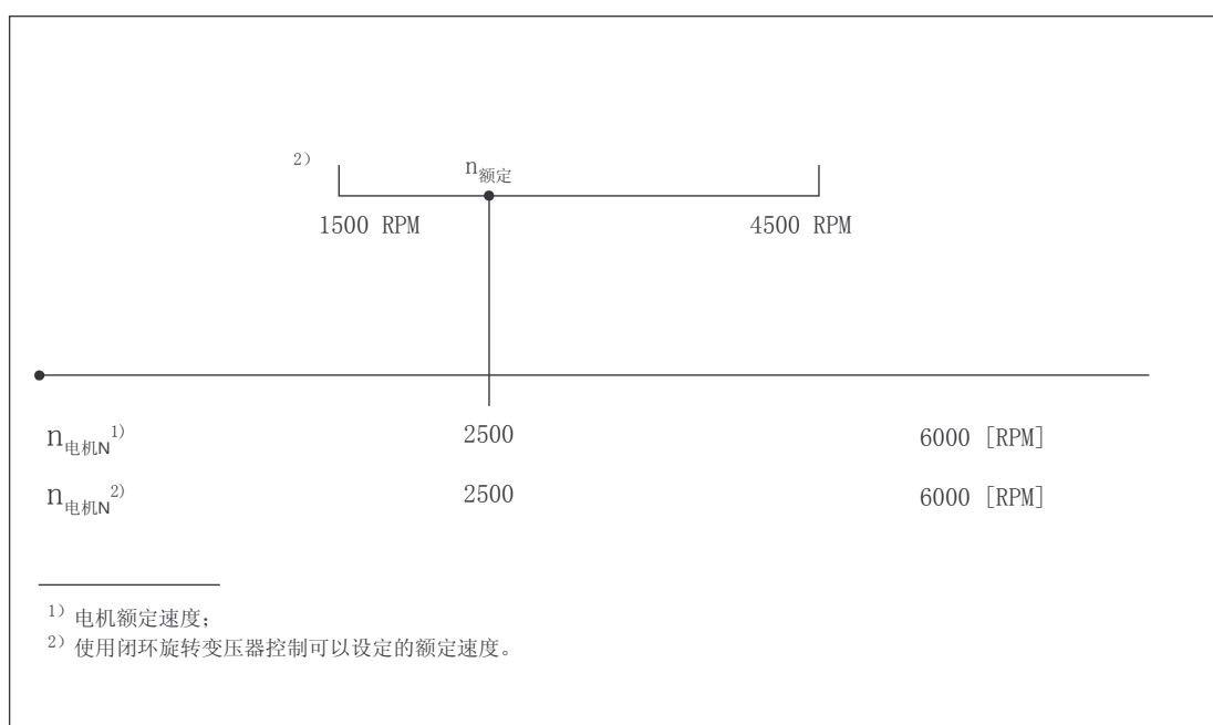
图2—6 \pm 10\text{V} 速度设定点的设定范围
