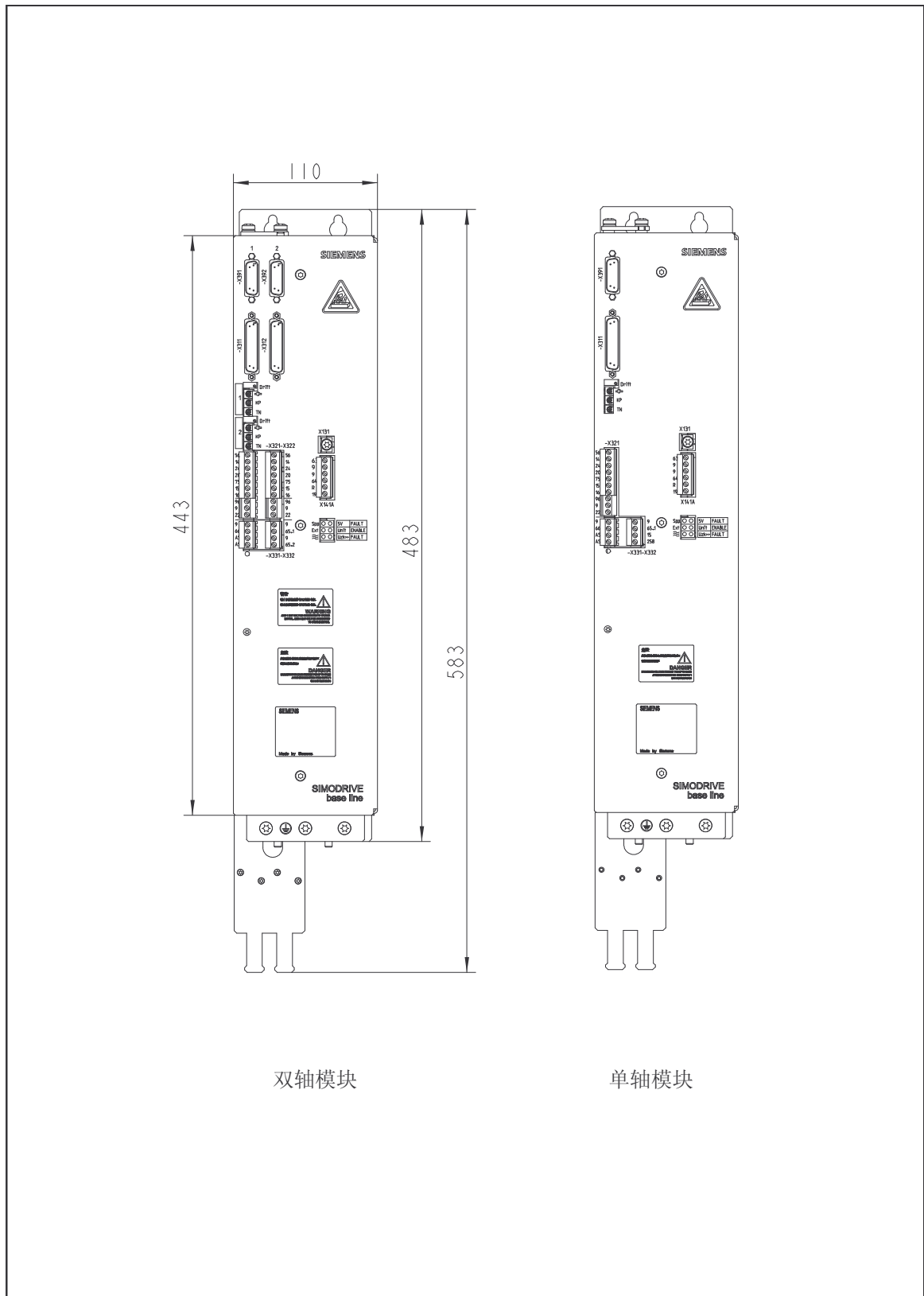
图2-2 安装尺寸 (续)
