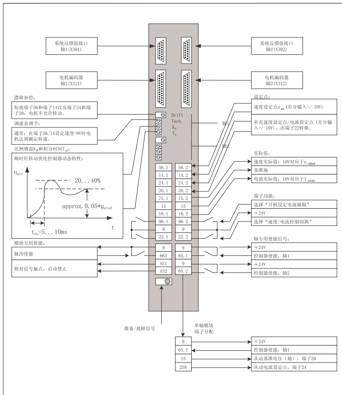
图2—5 控制模块接口（双轴伺服系统）
