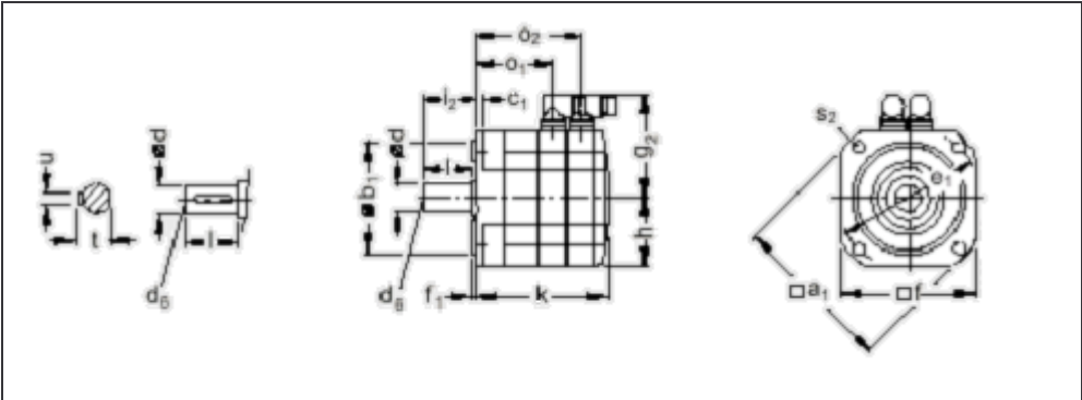
图4-5 电机尺寸图
