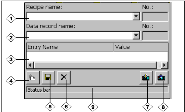
图7-5 配方视图的布局(实例)
