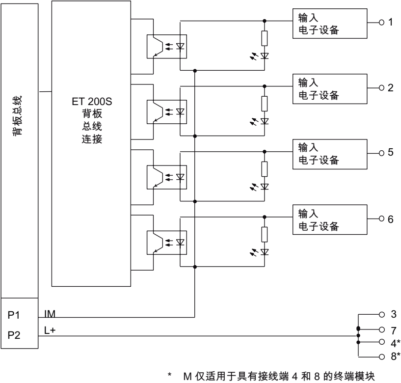
图 1-1 4DI DC24V ST 的方框图
