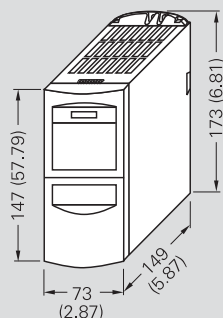
A 型外形尺寸变频器
