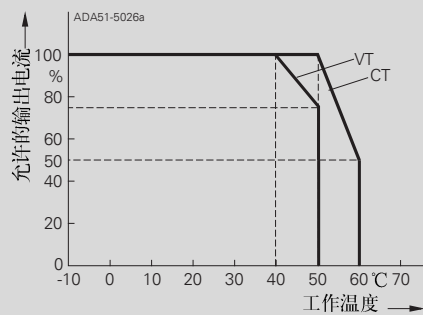
0.12 kW 至 75 kW 变频器
