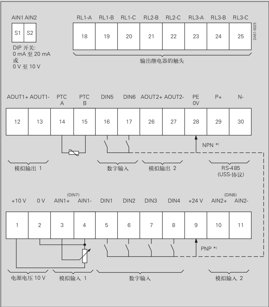
视图 A
