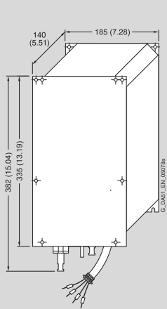
C 型变频器适用的 LC 滤波器
