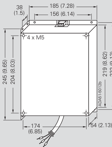
适合 C 型箱体尺寸的滤波器
