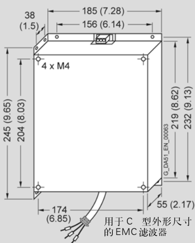
6SL3000- 型 A 级 EMC 滤波器
