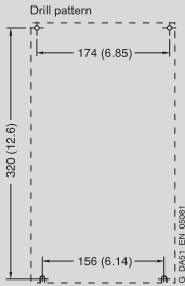
落地式安装, M5 螺栓
