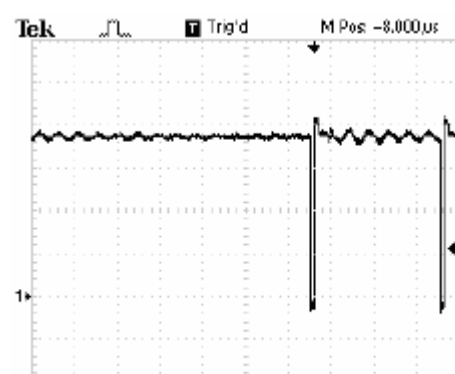
交流 220VAC，SW 脚电压波形
