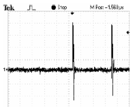
交流 220VAC，SW 脚电流波形
