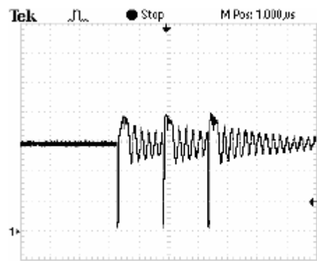
交流 220VAC，DRAIN 脚电流波形
