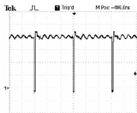
交流 110VAC，SW 脚电压波形
