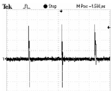
交流 110VAC，SW 脚电流波形
