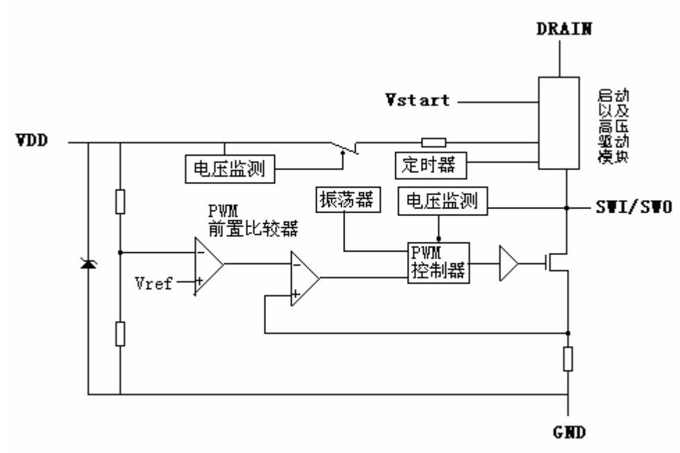
图一：芯片内部功能框图。
