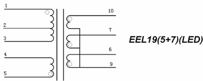
变压器原理图
