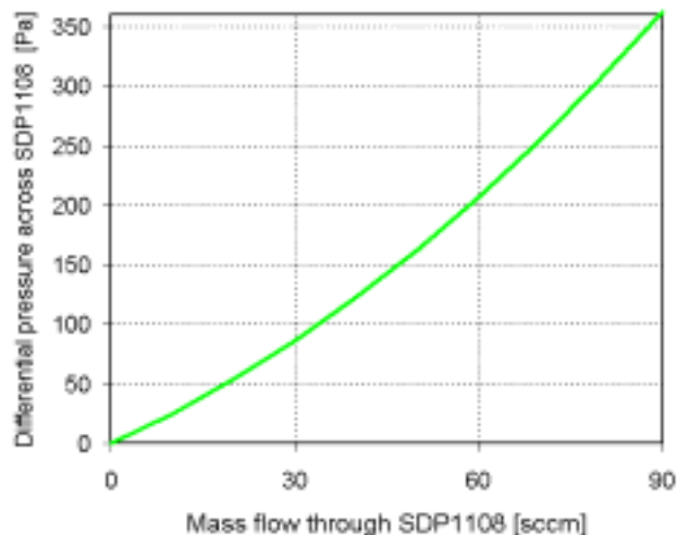
图 6: 通过 SDP1108 气体流量的典型值 i (注: 1 scc/min = 1 cm 3 /min at 0°C and 1013 mbar 压力(1 sccm = 0.001 标准公升))
