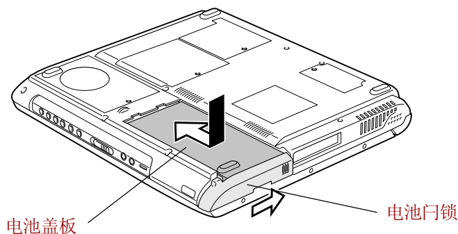
图6-4 固定电池组盖
