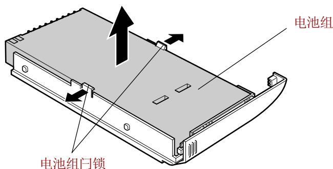
图6-2 取出电池组
