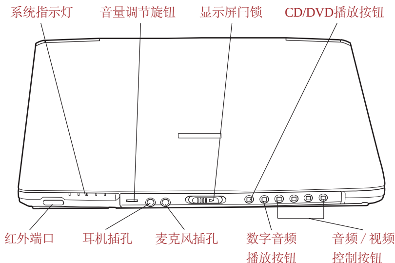
图2-1 电脑显示器关闭时的前侧
