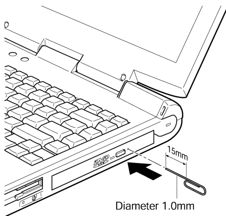
图4-3 使用弹出孔手工弹出托架
