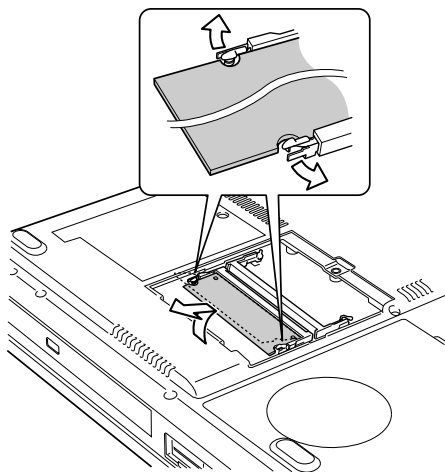
图8-7 拆除模块
