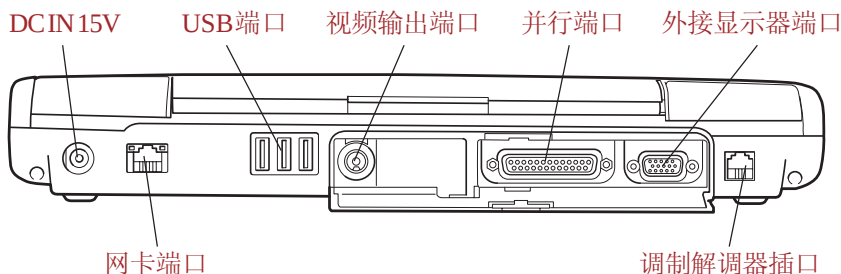
图2-4 电脑的后侧
