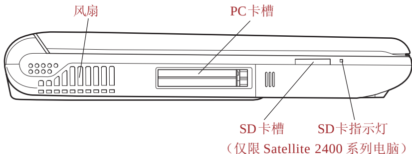
图2-2 电脑的左侧
