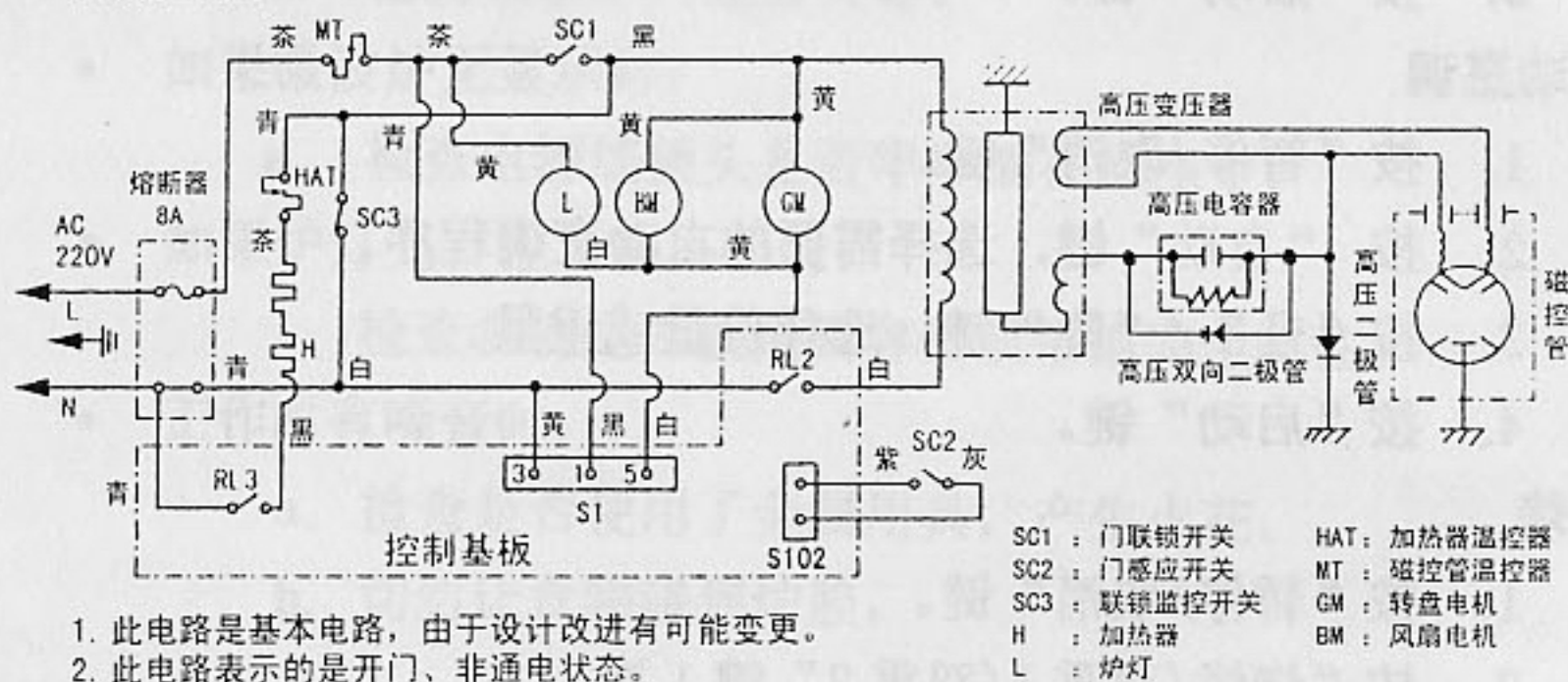
电路原理图
